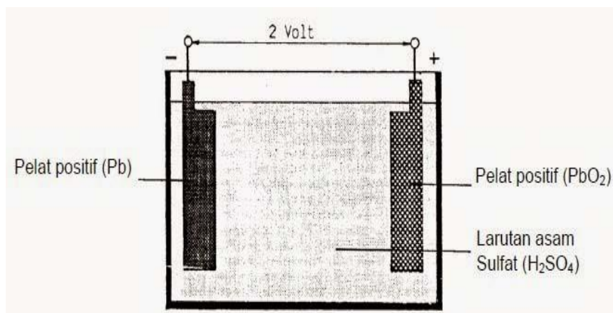
Gambar 2.8 Konstruksi Aki
