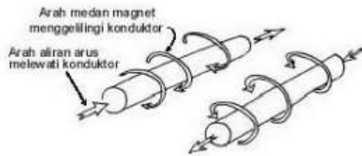
Gambar 2.17 Medan Magnet yang Membawa Arus pada Konduktor.
