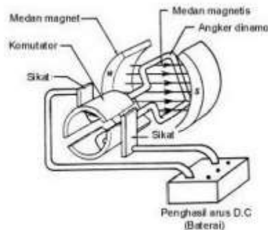
Gambar 2.16 Bagian Motor DC Sederhana
