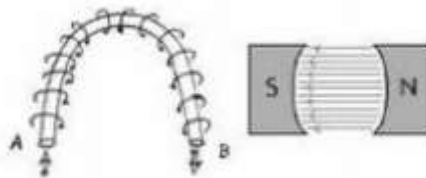
Gambar 2.18 Medan Magnet Mengeliling Konduktor dan diantara Kutub
