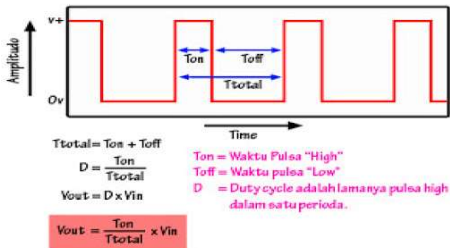
Gambar.2.10 sinyal PWM dan Perhitungannya
