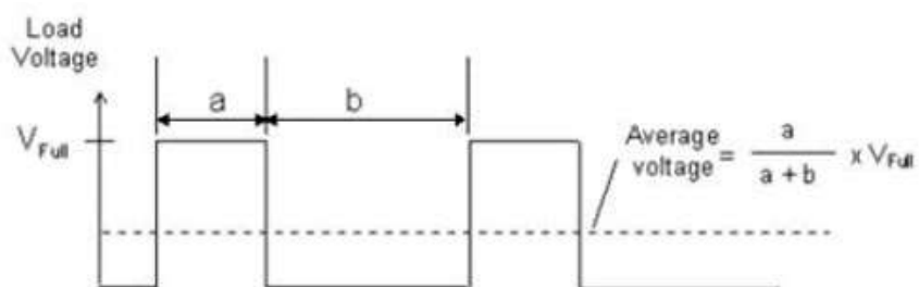
Gambar 2.12. Pengontrolan tegangan Pulsa
