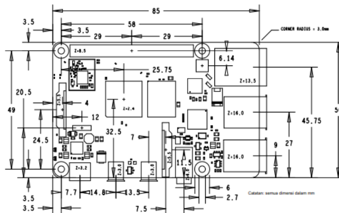
Gambar 2.6. Spesifikasi Fisik Raspberry PI 4
