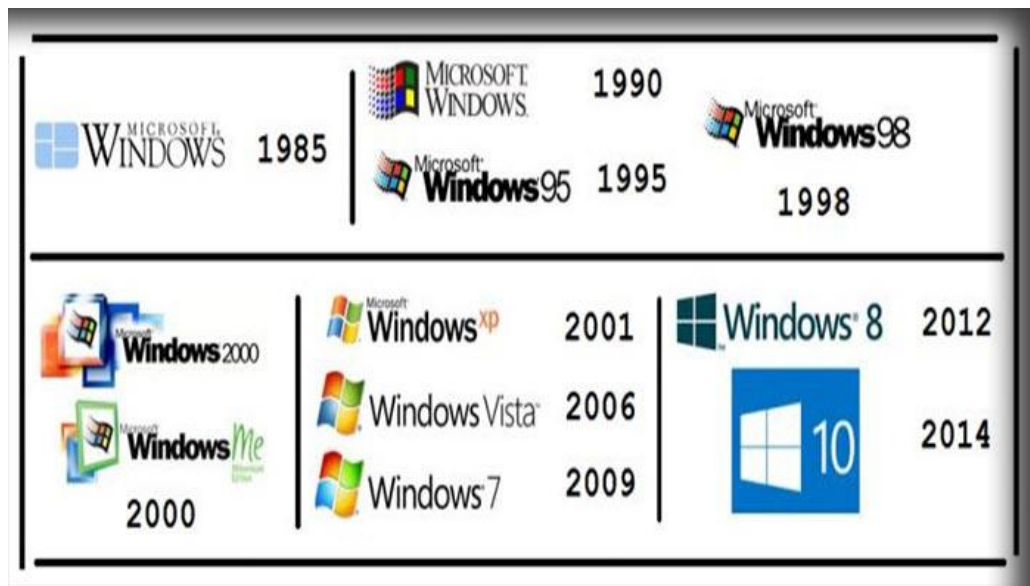
Gambar 2.12 Sejarah Windows
