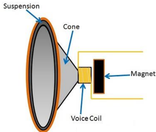
Gambar 2.7 Struktur Dasar Speaker
