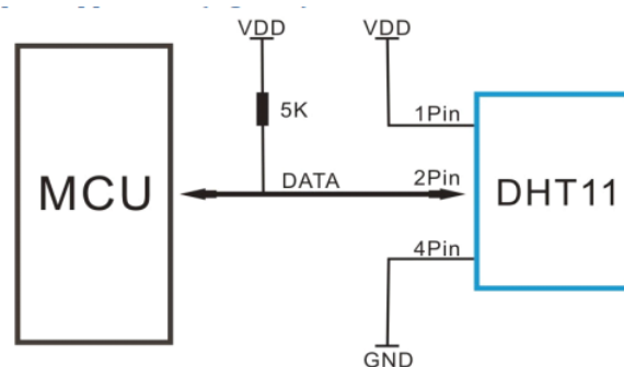
Gambar 2.7 Rangkaian Sensor suhu DHT11
