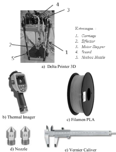
Gambar 4. Alat dan Bahan
