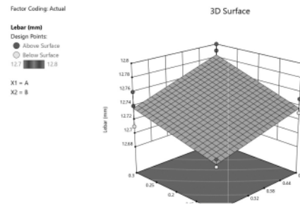
Gambar 8. Pengaruh Hubungan Antara Faktor Nozzle dan Tebal Lapisan Terhadap Respon Lebar.
