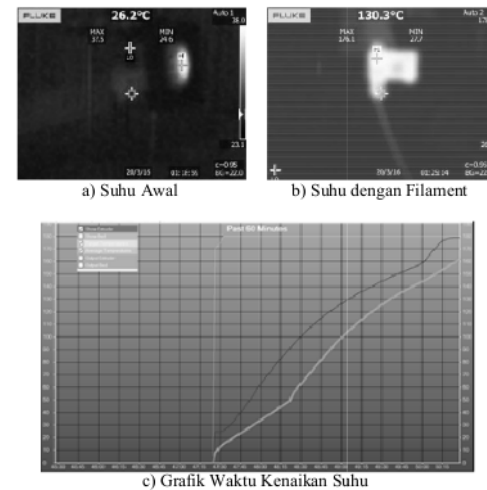
Gambar 5. Pengukuran Suhu Nozzle
