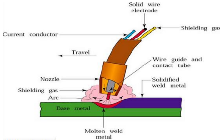
Gambar 2. 3 Pengelasan GMAW
