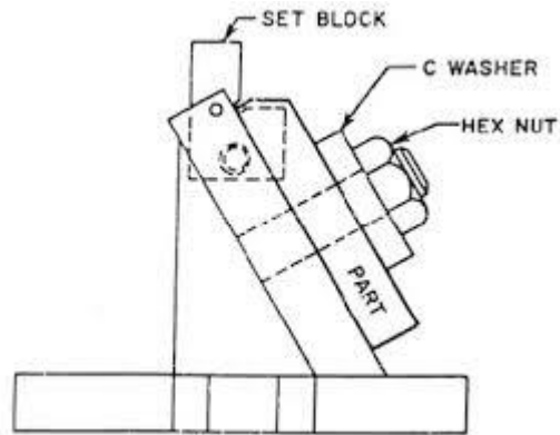
Gambar 2. 11 Fixture pelat sudut modifikasi
