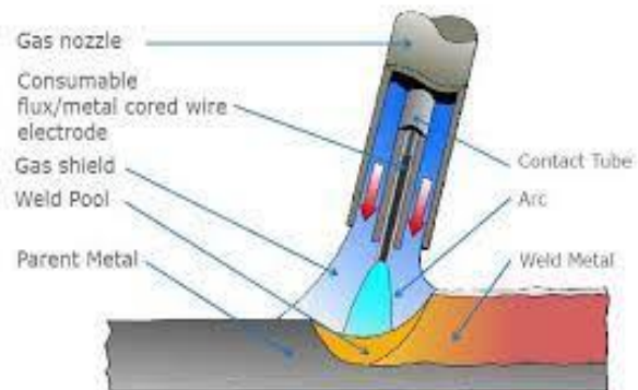
Gambar 2. 8 Pengelasan GTAW
