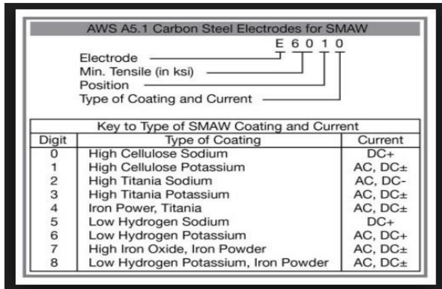
Gambar 2. 2 Kode Elektroda SMAW
