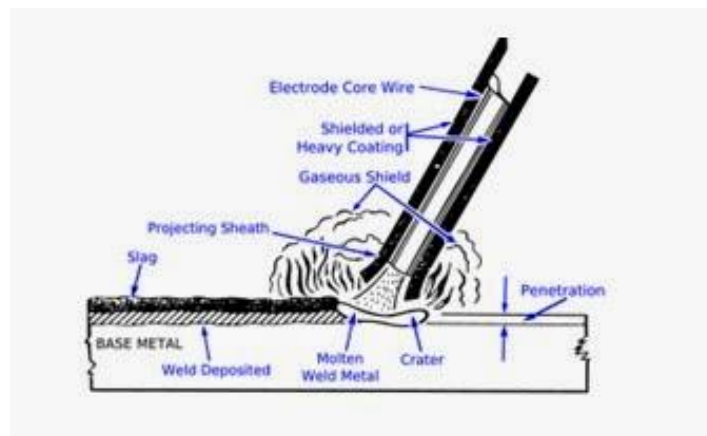
Gambar 2. 1 Pengelasan dengan SMAW
