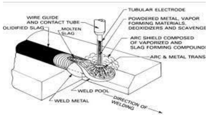
Gambar 2. 6 Pengelasan dengan FCAW
