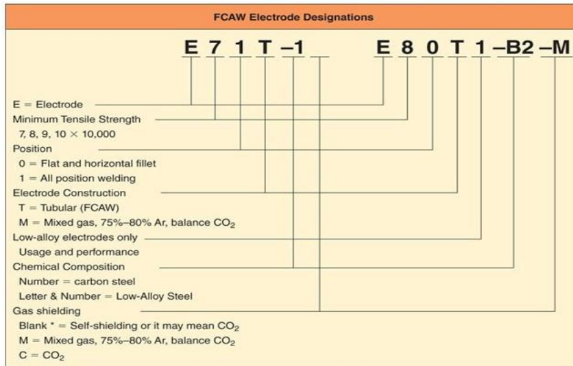
Gambar 2. 7 Kode elektroda FCAW
