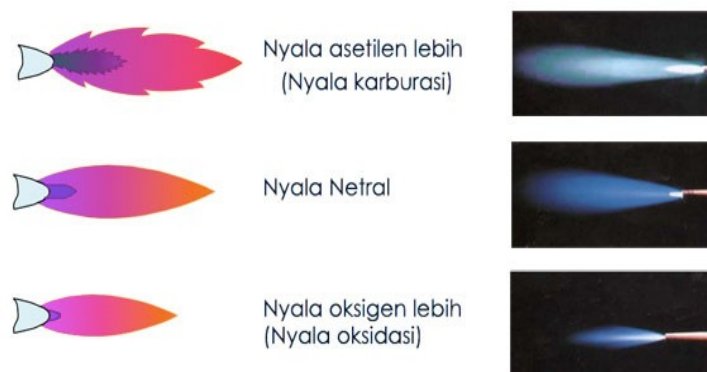
Gambar 2.39 Nyala Api Las Karbit
