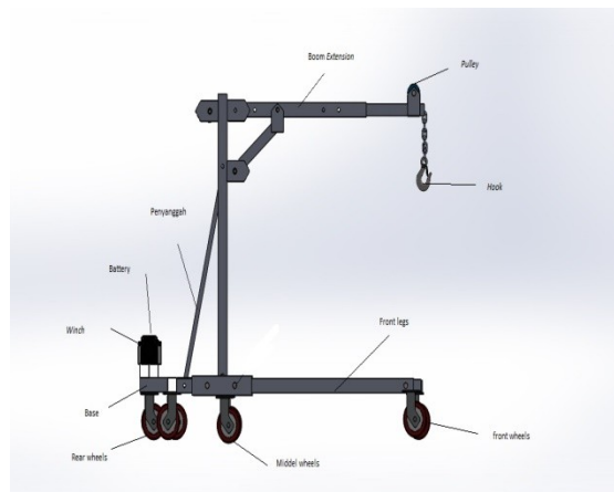
Gambar 2.1 Engine Crane (Sumber: Dokumentasi Pribadi)
