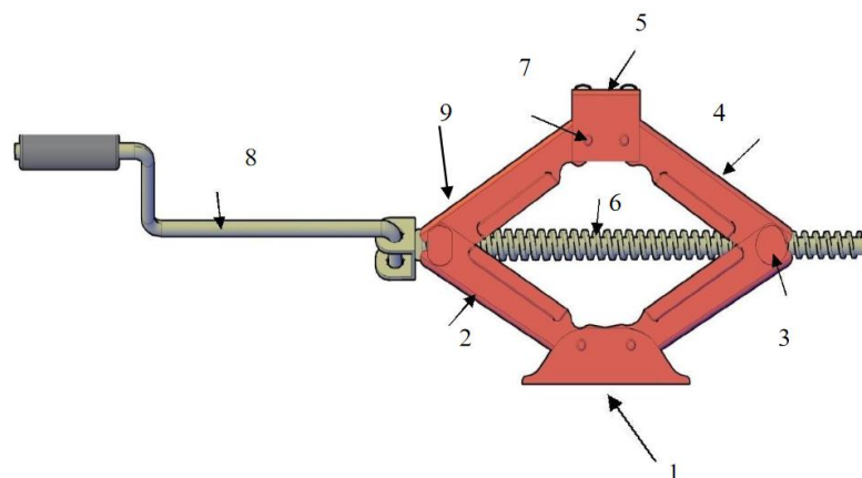
Gambar 2.11 Komponen Utama Dongkrak ulir [8]
