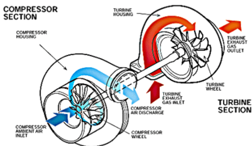
Gambar 2.7 Komponen Turbocharger [6]
