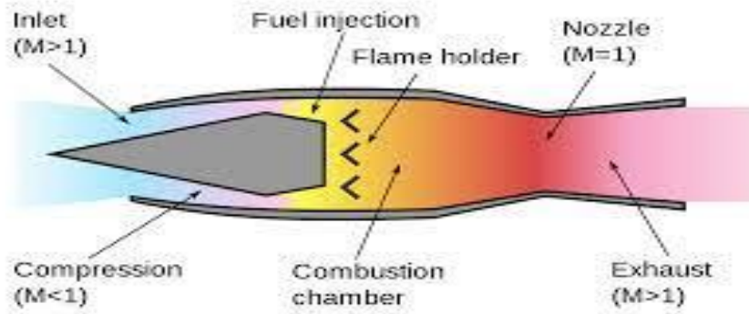
Gambar 2.2 Ramjet [2]
