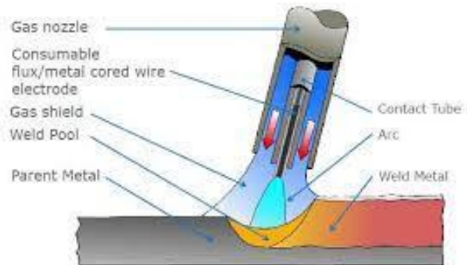
Gambar 2. 8 Pengelasan GTAW
