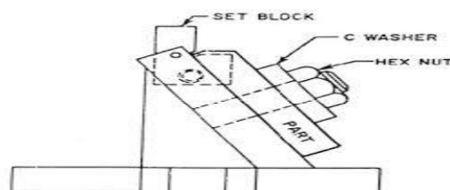
Gambar 2. 11 Fixture plat sudut modifikasi
