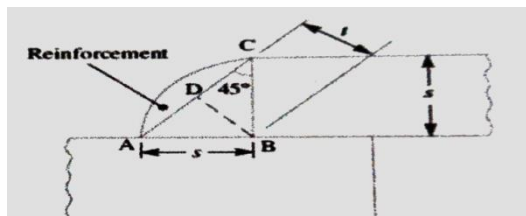
Gambar 2. 18 Tebal Las Sudut
