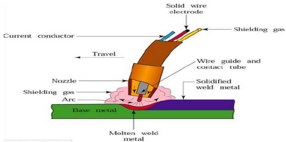
Gambar 2. 3 Pengelasan GMAW
