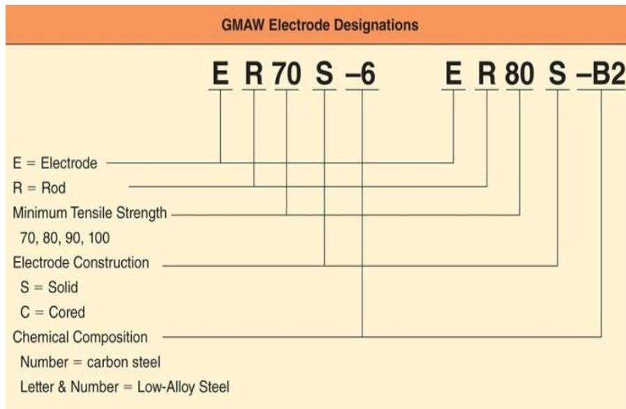
Gambar 2. 4 kode filler Metal GMAW
