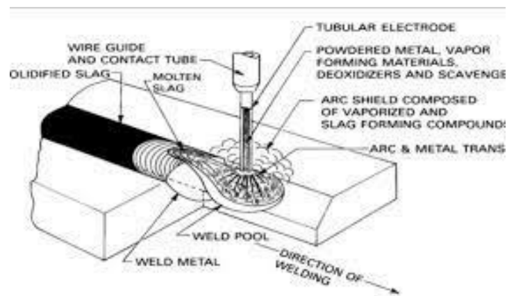
Gambar 2. 6 Pengelasan dengan FCAW
