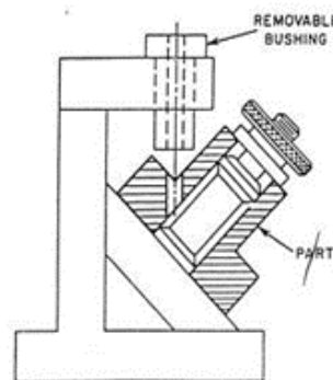
Gambar 2.12 Modifikasi Jig Angel Plate [23]
