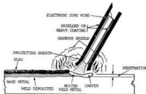
Gambar 2.0 Pengelasan dengan SMAW [10]
