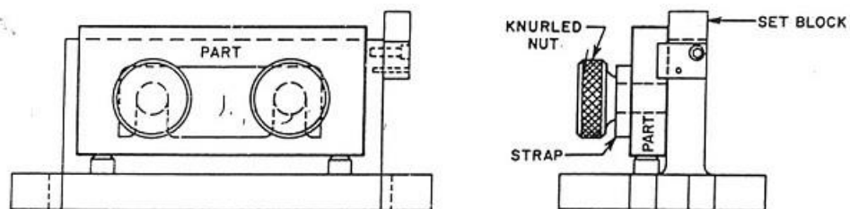
Gambar 2.21 Fixture pelat sudut [23]
