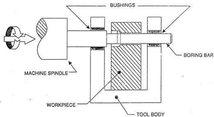
Gambar 2.6 Jig Bor [23]
