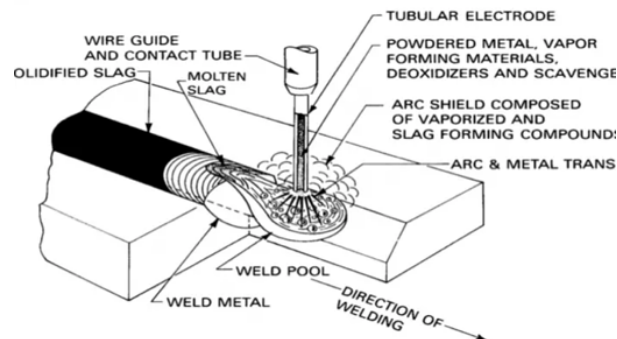
Gambar 2.3 Pengelasan dengan FCAW [2]
