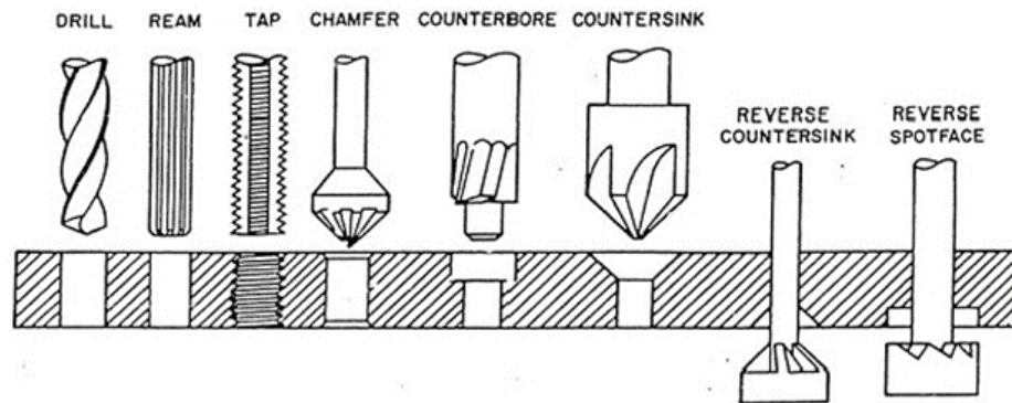
Gambar 2.7 Operasi umum Jig Gurdi [23]
