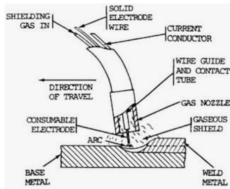
Gambar 2.1 Pengelasan dengan GMAW [9]
