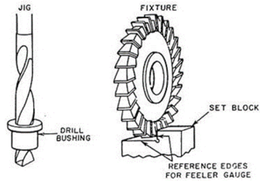
Gambar 2.5 Referensi alat bantu terhadap benda kerja [23]
