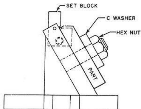
Gambar 2.22 Fixture pelat sudut modifikasi [23]
