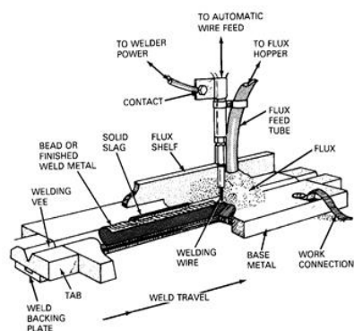
Gambar 2.2 Pengelasan dengan SAW [11]
