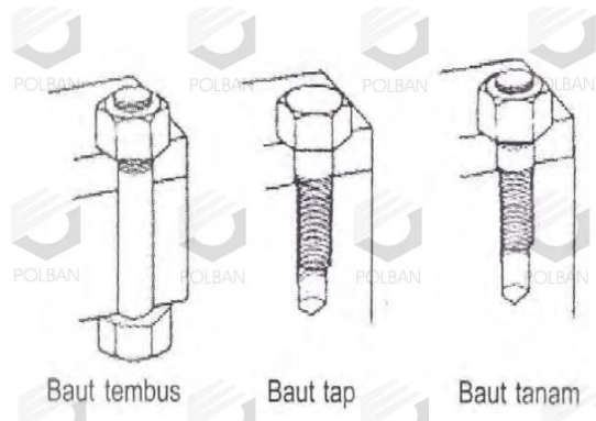
Gambar 2.32 Baut penjepit [4]
