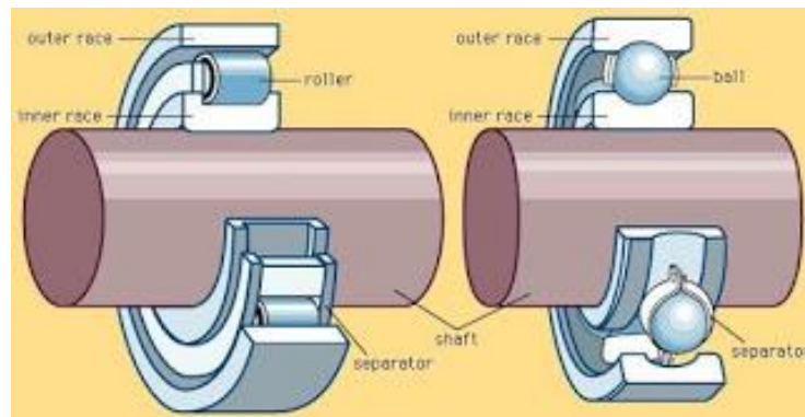
Gambar 2.28 Bearing atau Bantalan [12]
