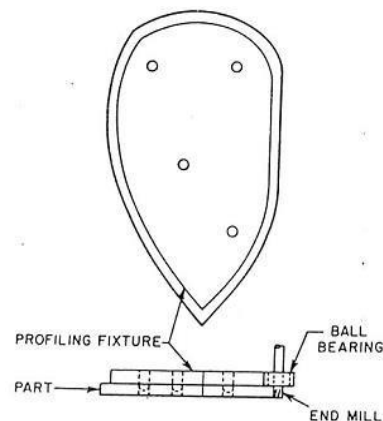
Gambar 2.27 Fixture profil [23]
