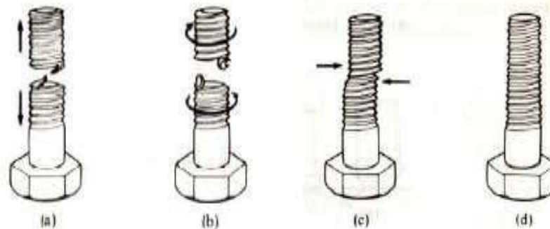
Gambar 2.31 Jenis – Jenis Kerusakann pada baut [21]
