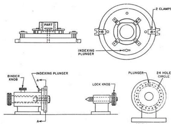
Gambar 2.25 Komponen mesin dengan menggunakan Fixture [23]
