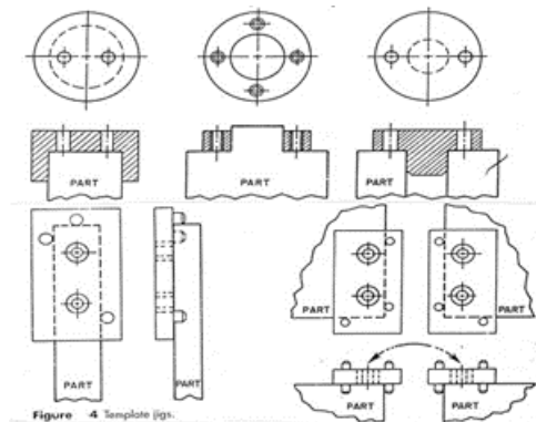
Gambar 2.8 Jig Template [23]
