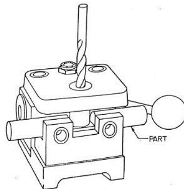
Gambar 2.18 Jig Pompa [23]
