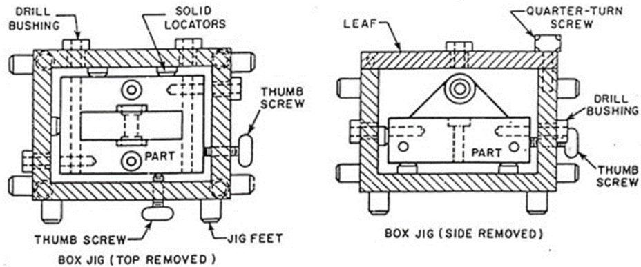
Gambar 2.13 Jig Kotak atau Tumble [23]
