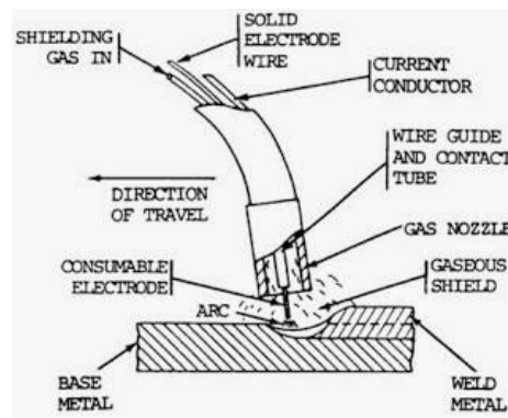
Gambar 2.2 Pengelasan dengan GMAW [3]
