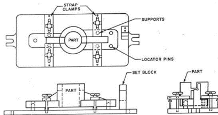
Gambar 2.21 Fixture Pelat [4]
