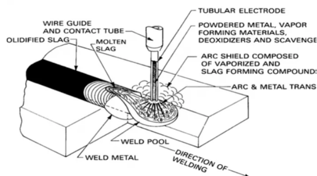
Gambar 2.4 Pengelasan dengan FCAW [3]
