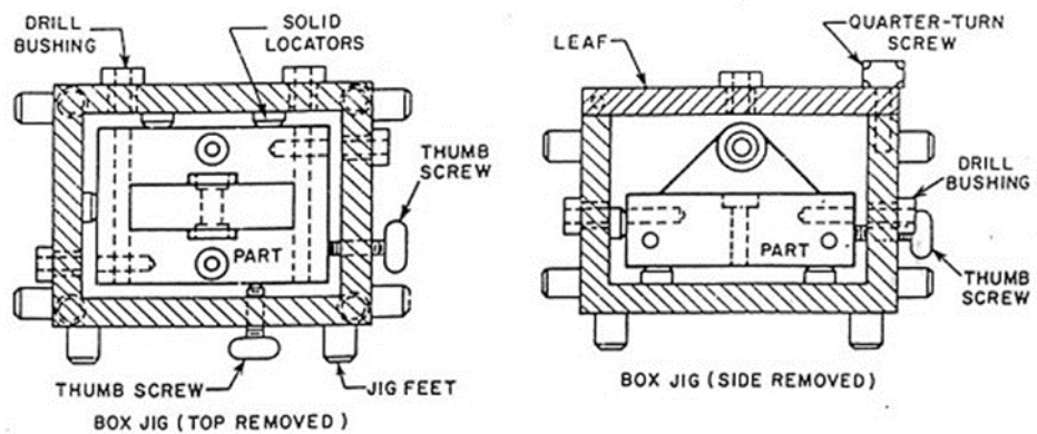
Gambar 2.14 Jig Kotak atau Tumble [5]
