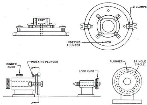
Gambar 2.26 Komponen mesin dengan menggunakan Fixture [4]
