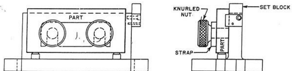
Gambar 2.22 Fixture pelatsudut [4]
