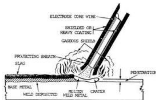
Gambar 2.1 Pengelasan dengan SMAW [3]
