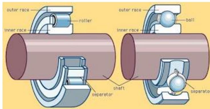
Gambar 2.29 Bearing atau Bantalan [8]
