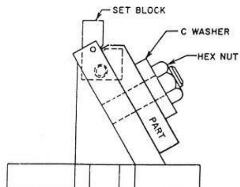
Gambar 2.23 Fixture pelat sudutmodifikasi [4]
