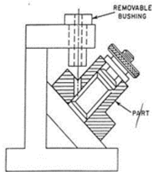
Gambar 2.13 Modifikasi Jig Angel Plate [5]
