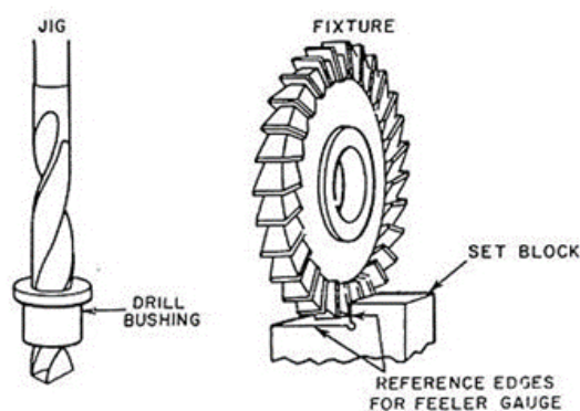
Gambar 2.6 Referensi alat bantu terhadap benda kerja [5]
