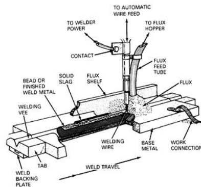
Gambar 2.3 Pengelasan dengan SAW [3]
