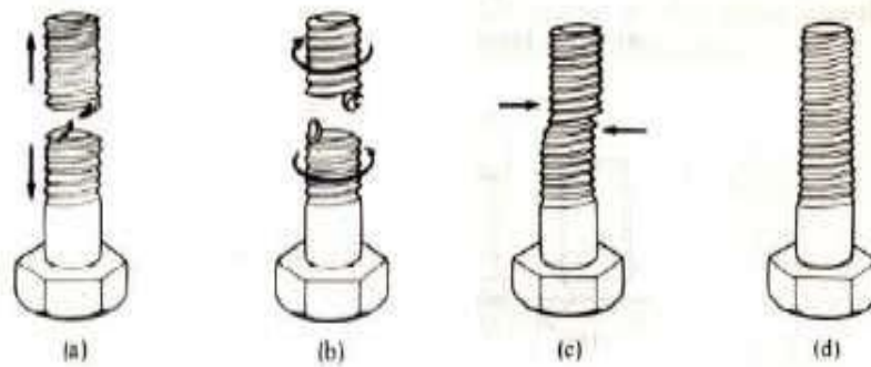
Gambar 2.32 Jenis – Jenis Kerusakann pada baut [8]
