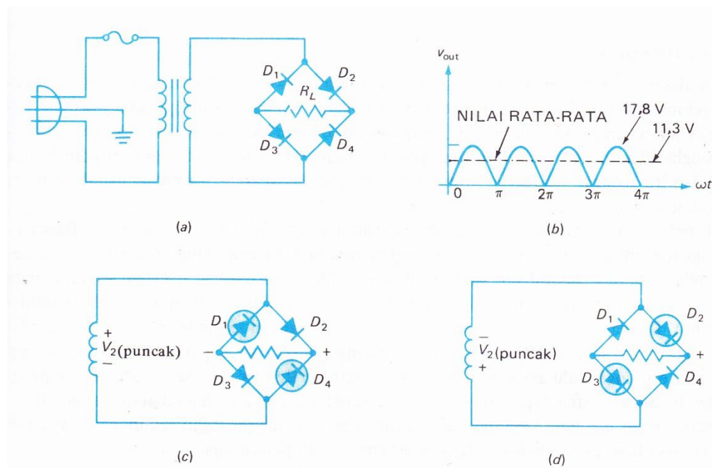
Gambar 2.4 (a). Penyearah Gelombang Penuh (b). Keluaran yang disearahkan (c). Setengah Siklus Positif (d). Setengah Siklus Negatif (Sumber : Malvino Barmawi Prinsip-Prinsip Elektronika 55)
