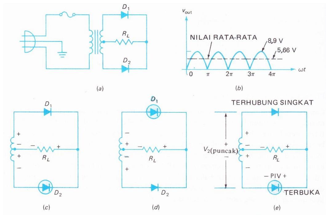
Gambar 2.3 (a). Penyearah Gelombang Penuh (b). Keluaran yang di Searahkan (c). Setengah Siklus Positif (d). Setengah Siklus Negatif (e). Pucak tegangan balik (Sumber : Malvino Barmawi Prinsip-Prinsip Elektronika 52)
