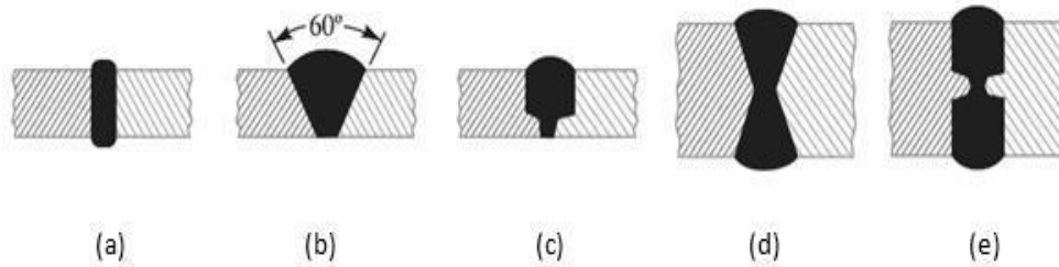
Gambar 2.16 Bentuk alur / kempuh las
