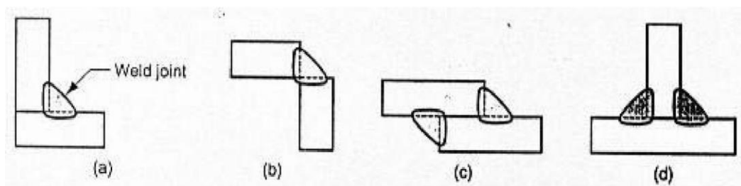
Gambar 2.15 Jenis sambungan las
