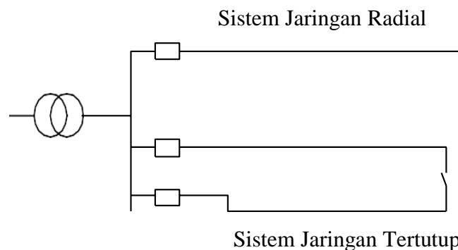
Gambar 2.4 Pola Jaringan Distribusi Dasar.
