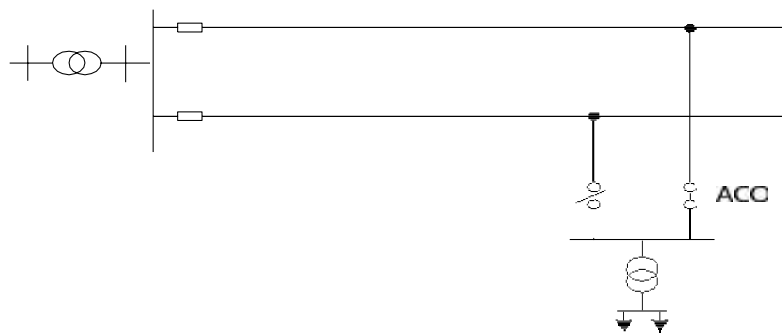
Gambar 2.8 Konfigurasi Fork
