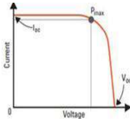
Gambar 2.9 Gambar Kurva arus dan tegangan
