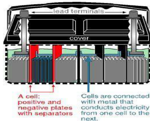
Gambar 2.17 Gambar Struktur Konstruksi Baterai Deep Cycle
