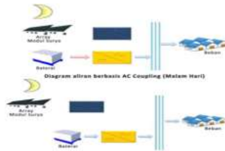
Gambar 2. 5 Gambar Aliran Energi pada Malam Hari
