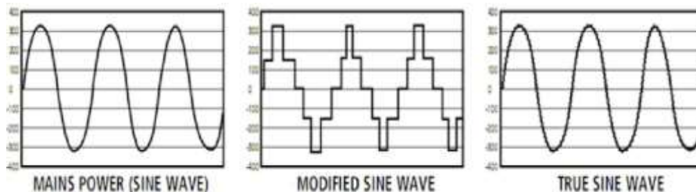
Gambar 2.13 Gambar Bentuk Gelombang Inverter
