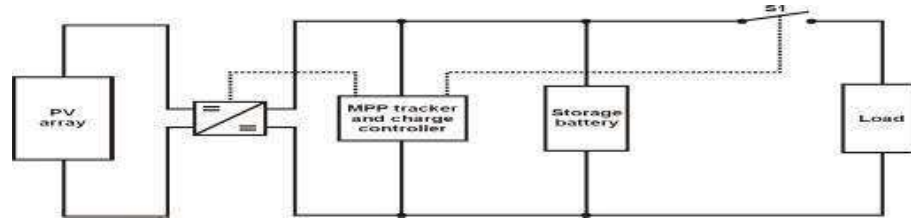
Gambar 2.15 Gambar Rangkaian MPP Tracker dan Charge Control PV Array
