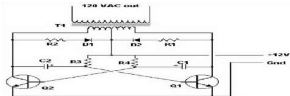
Gambar 2.12 Gambar Rangkaian dasar sederhana inverter
