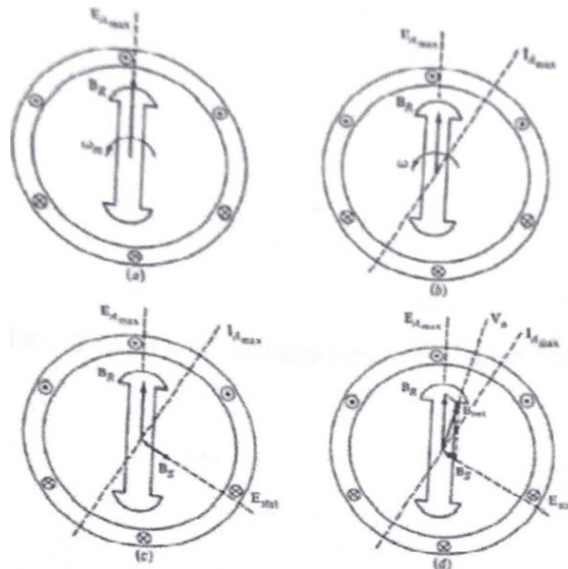
Gambar 2.7 Reaksi Jangkar 6
