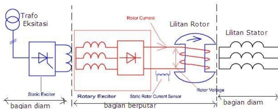
Gambar 2.17 Sistem Eksitasi Tanpa Sikat (Brushless Excitation) 9
