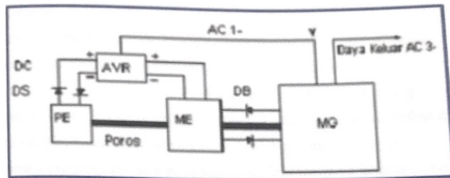
Gambar 2.18 Cara Kerja Eksitasi Tanpa Sikat 10
