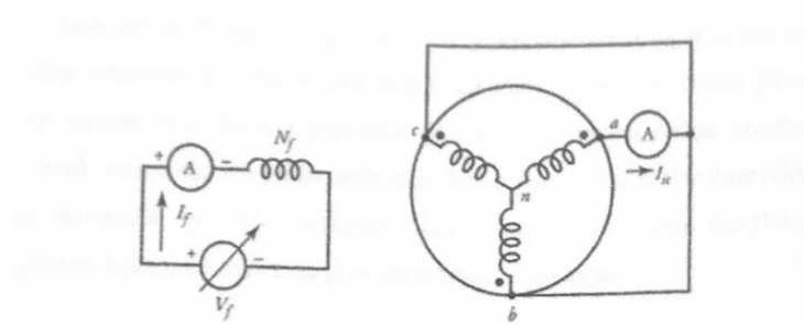
Gambar 2.15 Rangkaian Tes Short Circuit
