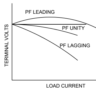
Gambar 2.11 Karakteristik Generator AC pada Berbagai Faktor Daya
