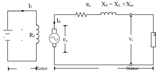
Gambar 2.10 Rangkaian Ekuivalen Generator Sinkron Berbeban.
