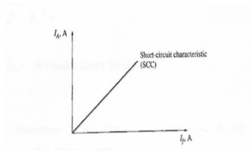
Gambar 2.14 Karakteristik Hubung Singkat Generator Sinkron
