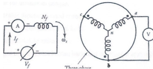
Gambar 2.12 Circuit Diagram Tes Rangkaian Terbuka
