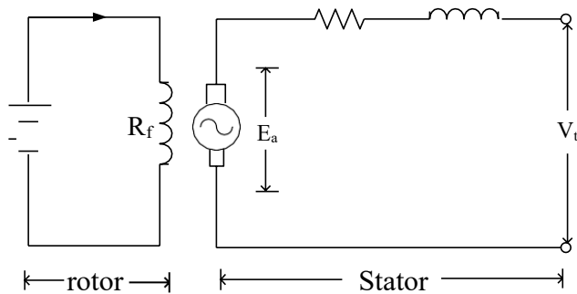
Gambar 2.8 Rangkaian Ekuivalen Generator Sinkron Tanpa Beban
