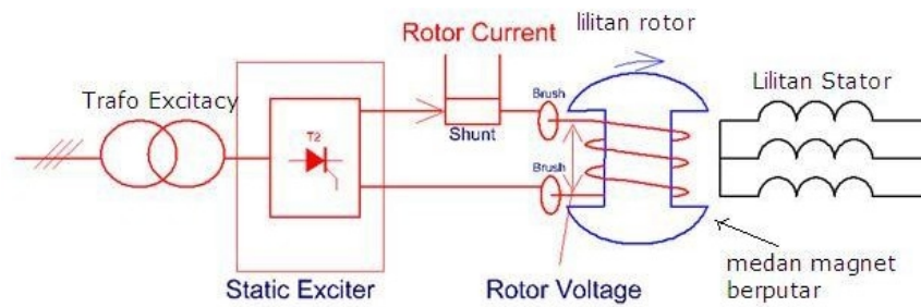
Gambar 2.16 Sistem Eksitasi Menggunakan Sikat (Brushless Excitation) 8
