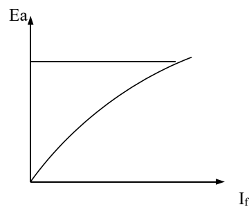
Gambar 2.9 Grafik Hubungan Arus Penguat Medan ( I_f ) dan E_a
