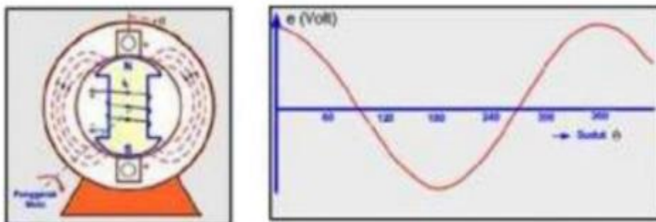
Gambar 2.12 Diagram Generator AC Satu Fasa Dua Kutub
