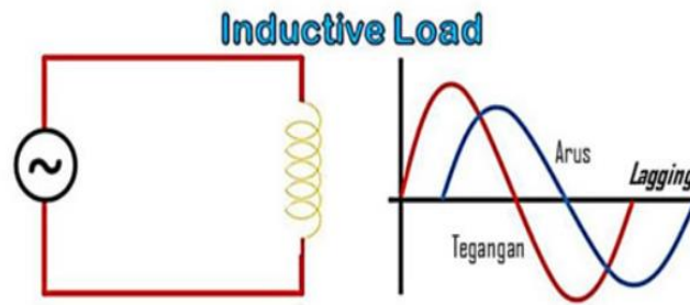
Gambar 2.18 Rangkaian Beban Induktif beserta Gelombang AC
