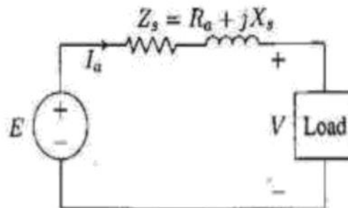
Gambar 2.11 Rangkaian Ekuivalen pada Generator Sinkron
