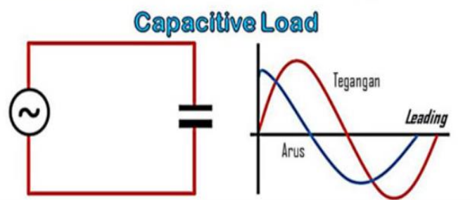
Gambar 2.20 Rangkaian Beban Kapasitif beserta Gelombang AC
