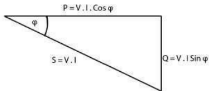
Gambar 2.1 Segitiga Daya
