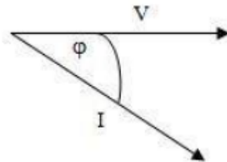
Gambar 2.19 Grafik Arus dan Tegangan Pada Beban Induktif
