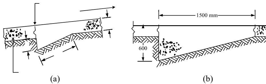
(Sumber: Perencanaan Perkerasan Jalan Beton Semen, 2003) Gambar 2.41 (a) Angker Panel dan (b) Angker Blok
