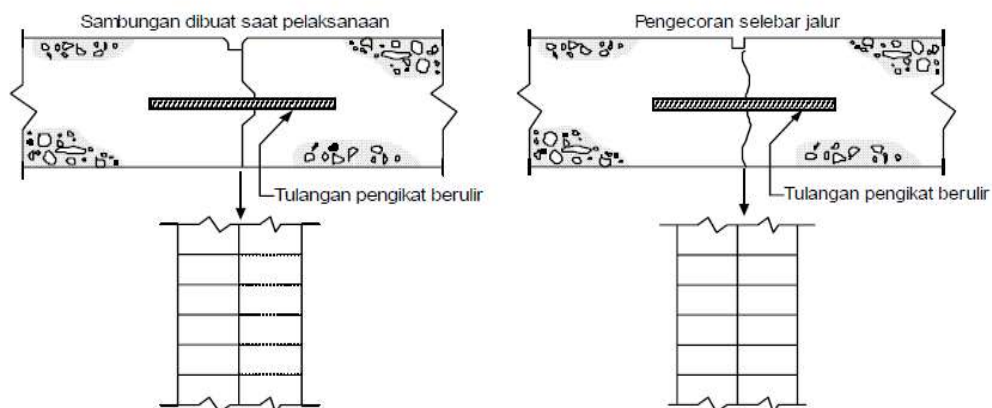
Gambar 2.32 Tipikal Sambungan Memanjang
