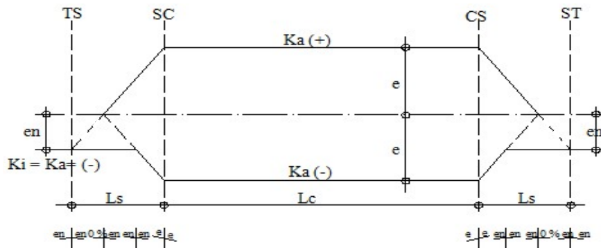
Gambar 2.18 Diagram Superelevasi Spiral - Circle - Spiral (Sumber : Shirley L. Hendarsin, dalam Perencanaan Teknik Jalan Raya, 2000)
