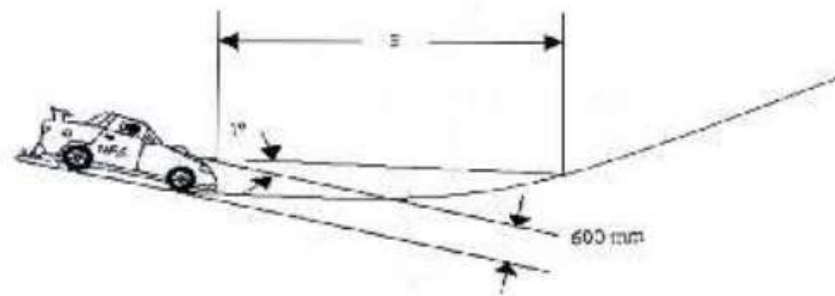
Gambar 2.24 Asumsi penentuan Panjang Lengkung Vertikal Cekung
