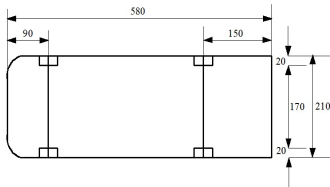
Gambar 2.2 Dimensi Kendaraan Kecil
