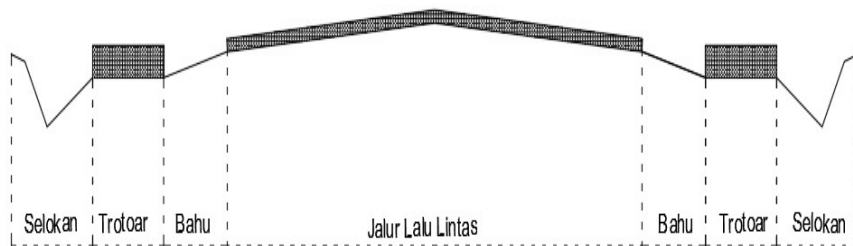
Gambar 2.7 Penampang Melintang Jalan Tipikal dilengkapi trottoar
