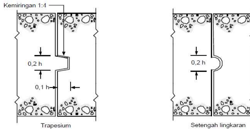
Gambar 2.33 Ukuran Standar Penguncian Sambungan Memanjang
