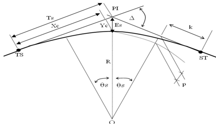
Gambar 2.16 Tikungan Spiral - Spiral (SS) (Sumber : Shirley L. Hendarsin, dalam Perencanaan Teknik Jalan Raya, 2000)
