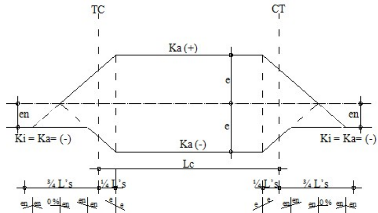
Gambar 2.17 Diagram Superelevasi Full Circle (Sumber : Shirley L. Hendarsin, dalam Perencanaan Teknik Jalan Raya, 2000)
