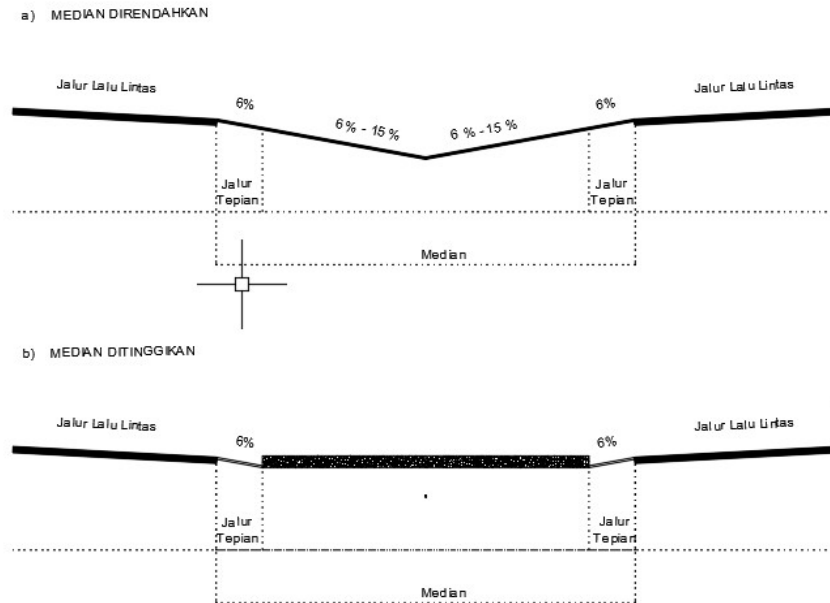
Gambar 2.10 Median direndahkan dan ditinggikan
