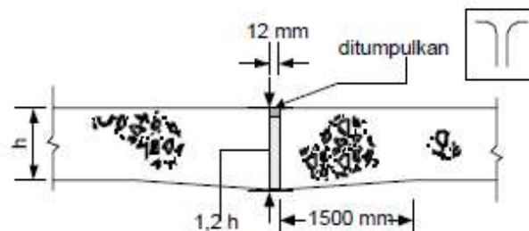
Gambar 2.37 Sambungan isolasi dengan ruji
