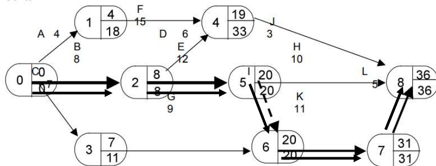
(Sumber : Penguasaan Metode Diagram Panah Sebagai Langkah Awal Pemahaman Terhadap Dasar-Dasar Penyusunan Network Planning Metoda Jalur Kritis/Sumardjito/Hal 153) Gambar 2.44 Sketsa Network planning
