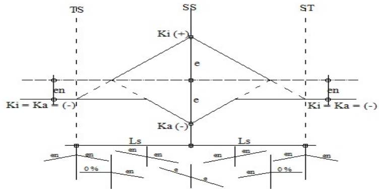
Gambar 2.19 Diagram Superelevasi Spiral - Spiral (Sumber : Shirley L. Hendarsin, dalam Perencanaan Teknik Jalan Raya, 2000)
