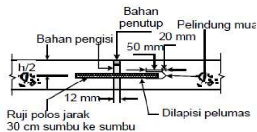
Gambar 2.37 Sambungan isolasi dengan ruji
