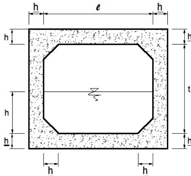
Gambar 2.43 Sketsa Box Culvert dengan Bentuk persegi
