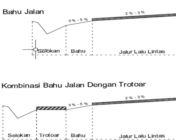
Gambar 2.9 Bahu Jalan
