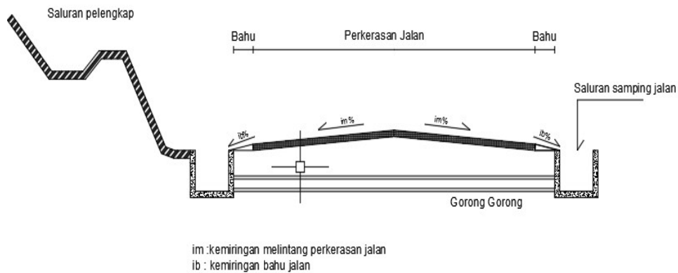
Gambar 2.8 Kemiringan Melintang Jalan Normal
