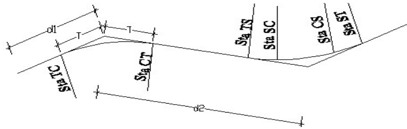
Gambar 2.21 Sistem Penomoran Stationing Jalan
