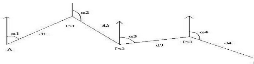
Gambar 2.12 Sudut Jurusan ( \alpha )
