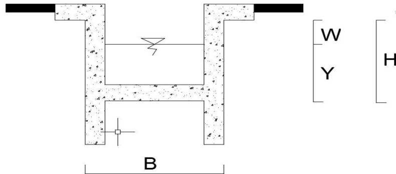
Gambar 2.42 Sketsa saluran dengan bentuk persegi
