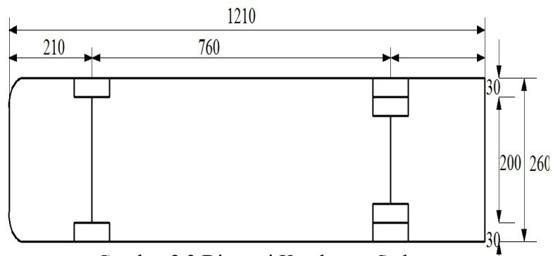
Gambar 2.3 Dimensi Kendaraan Sedang
