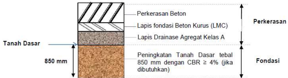
Gambar 2.27 Gambar tipikal perkerasan kaku pada timbunan
