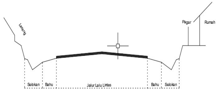
Gambar 2.6 Penampang Melintang Jalan Tipikal
