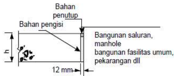
Gambar 2.38 Sambungan isolasi dengan penebal tepi
