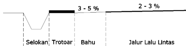
Gambar 2.7 Bahu Jalan
