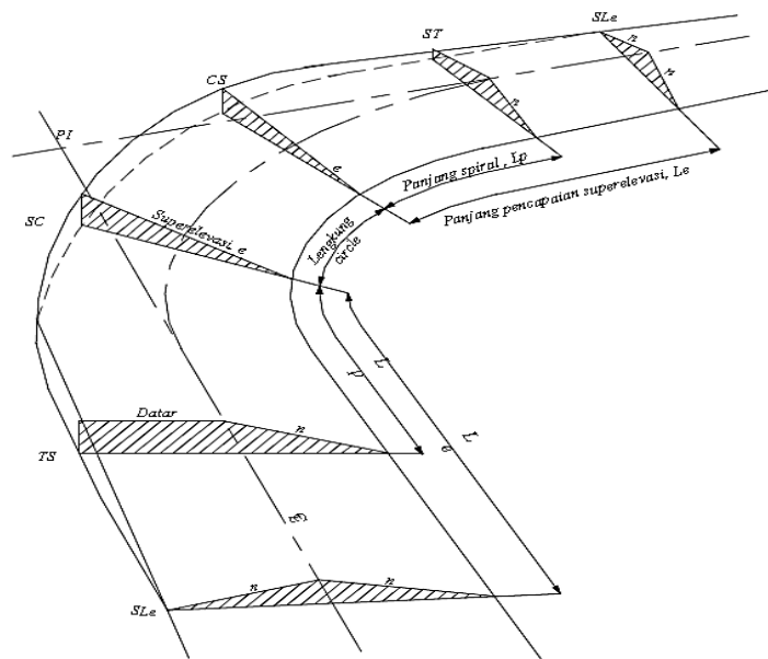
Gambar 2.14 Perubahan Superelevasi
