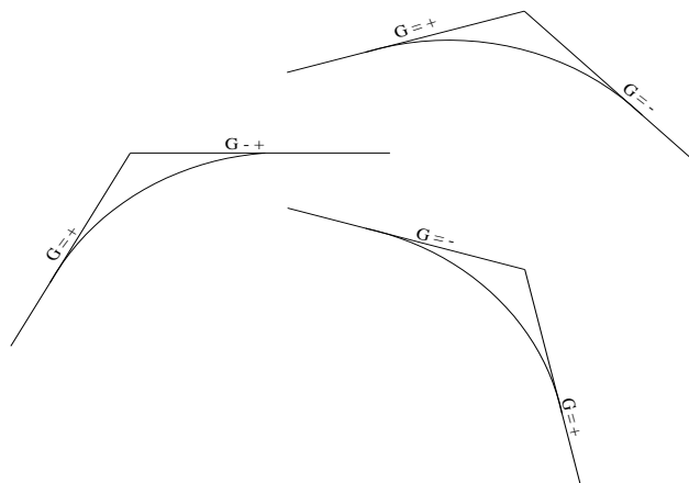
Gambar 2.27 Alinyemen Vertikal Cembung
