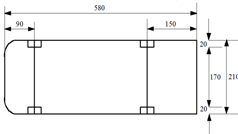
Gambar 2.2 Dimensi Kendaraan Kecil
