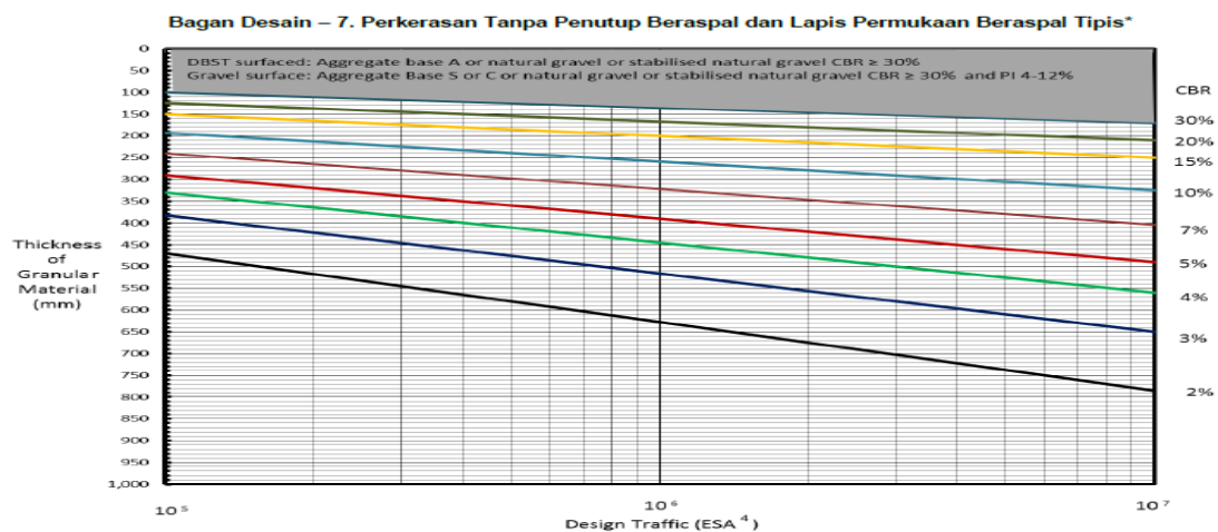
Gambar 3.71 Gafik Desain Perkerasan Tanpa Penutup Beraspal Dan Lapis Permukaan Beraspal Lapis
