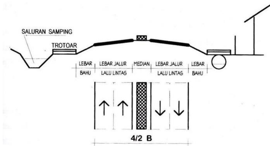
Gambar 2.2 Penampang Melintang Jalan dengan Median
