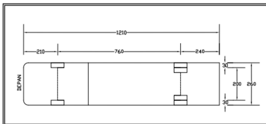
Gambar 2.5 Dimensi Kendaraan Sedang
