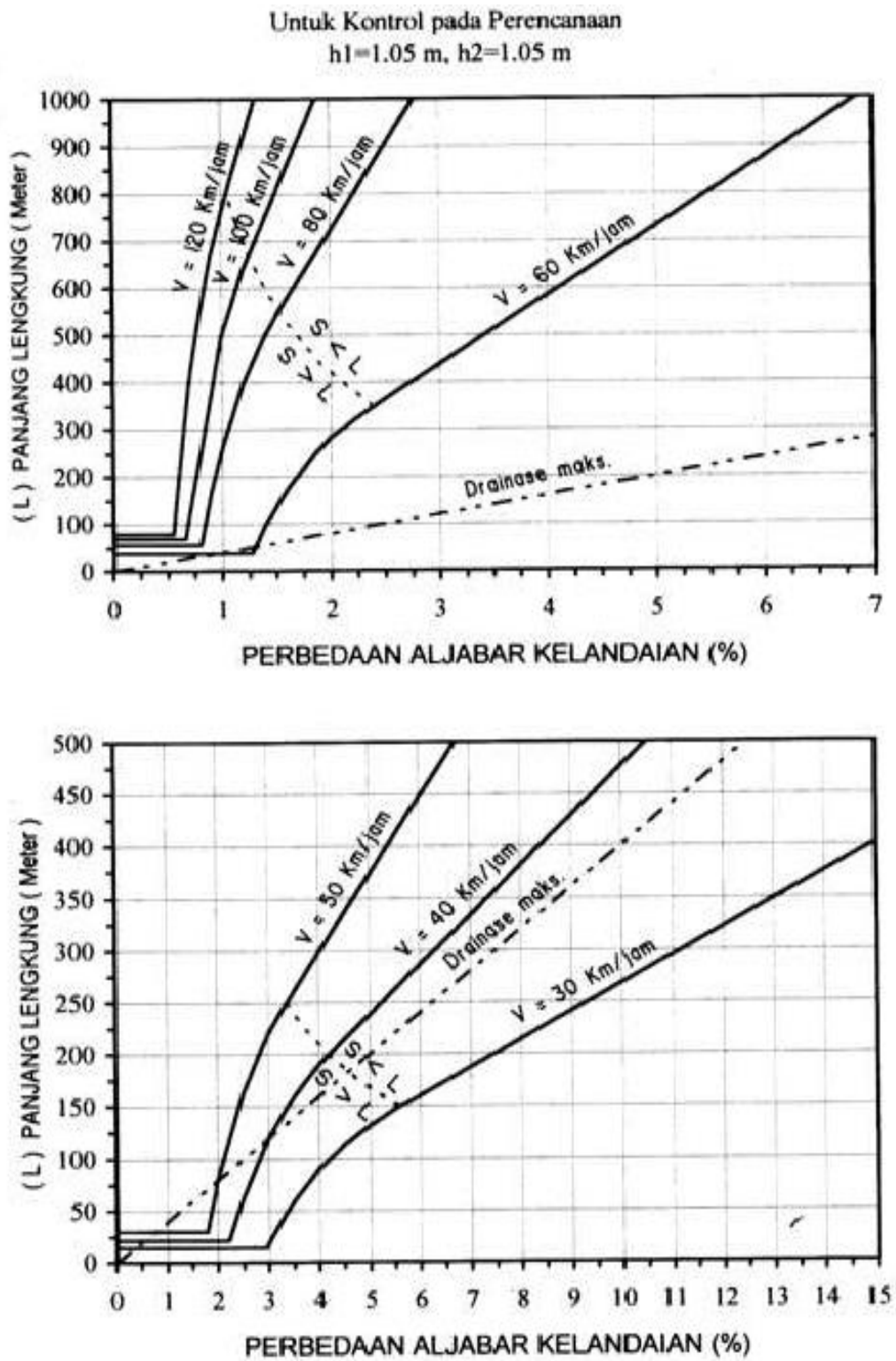
Gambar 2.32 Jarak Pandang Mendahului (Jd)
