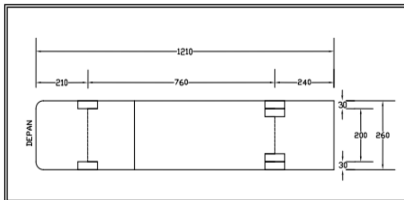
Gambar 2.6 Dimensi Kendaraan Besar
