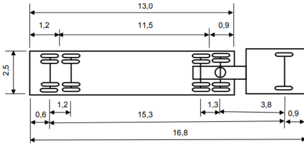
Gambar 2.13 Kendaraan Semitrailer Kombinasi Besar (WB-15)
