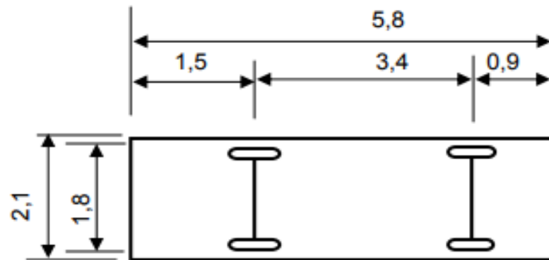
Gambar 2.7 Kendaraan Penumpang (P)
