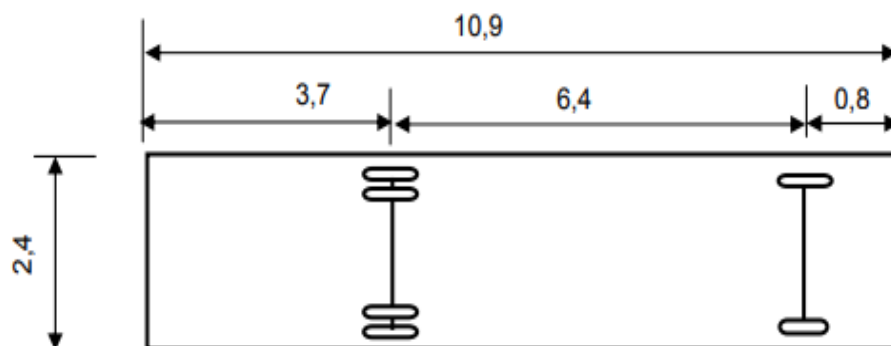
Gambar 2.9 Kendaraan Bus Sekolah (SB)
