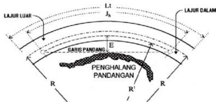
Gambar 2.25 Daerah bebas samping ditikungan untuk J_h > L_t
