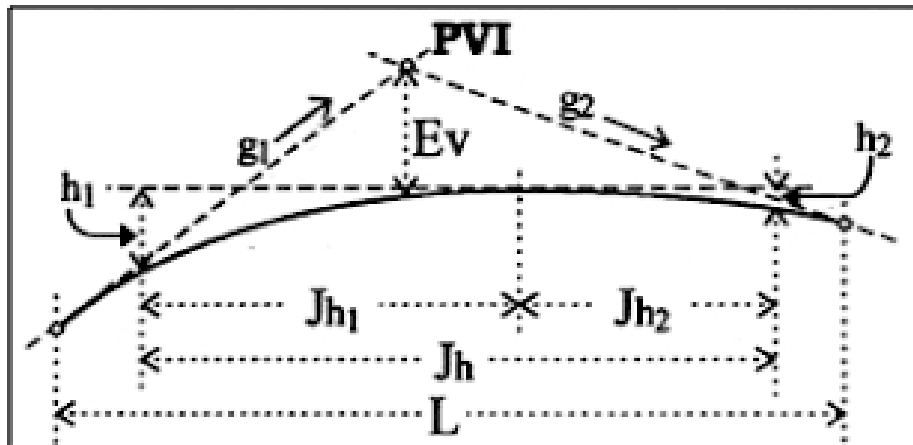
Gambar 2.29 Panjang Lv untuk J_h < L_v
