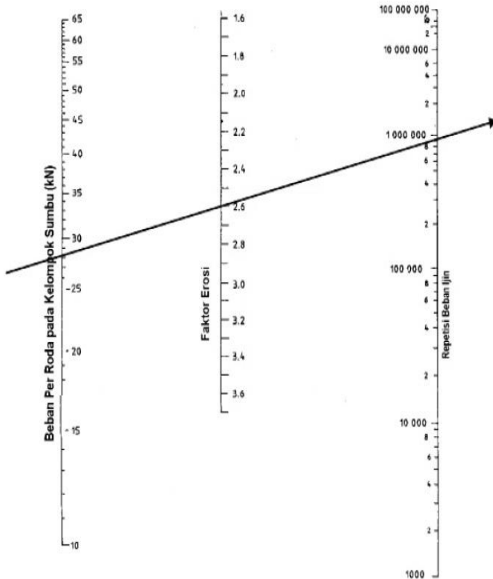
Gambar 2.42 Analisis Erosi dan Jumlah Repetisi Beban Ijin, Berdasarkan Faktor Erosi, dengan Bahu Beton
