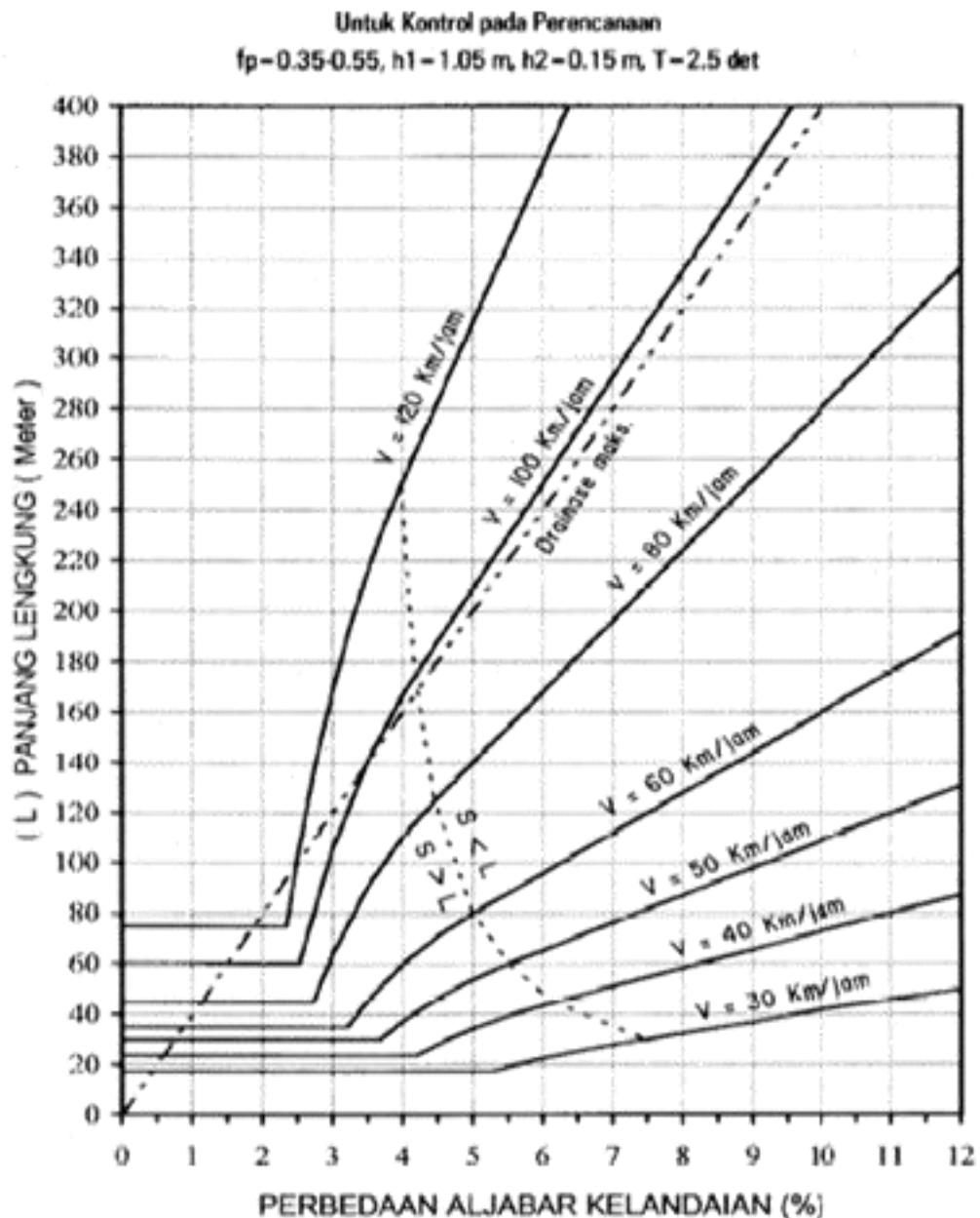
Gambar 2.34 Grafik Panjang Lengkung Vertikal Cekung
