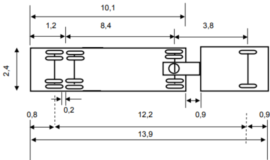
Gambar 2.12 Kendaraan Semitrailer Kombinasi Sedang (WB-12)
