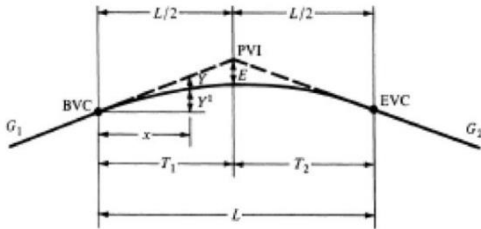
Gambar 2.27 Lengkung Vertikal
