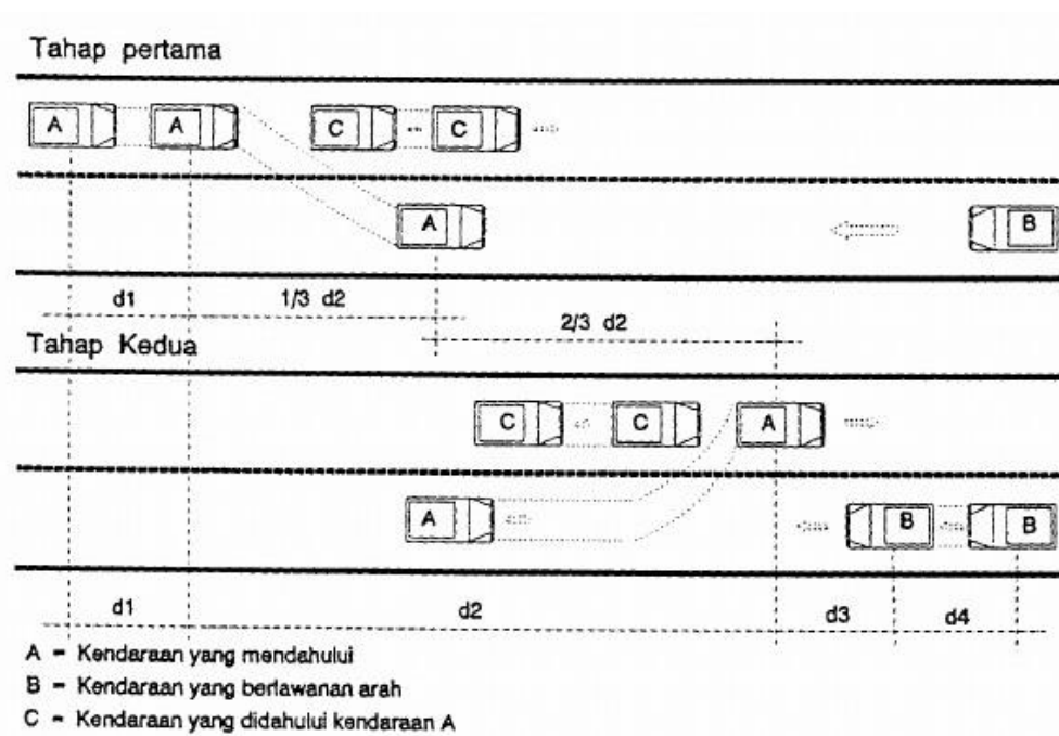
Gambar 2.16 Diagram Pergerakan Kendaraan Untuk Mendahului
