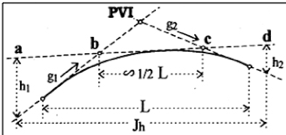
Gambar 2.30 Panjang Lv untuk J_h > L_v
