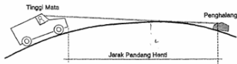
Gambar 2.14 Jarak Pandang Henti pada Lengkung Vertikal Cembung
