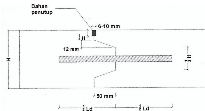
Gambar 2.44 Sambungan Pelaksanaan Memanjang dengan Lidah Alur Dan Tie Bar
