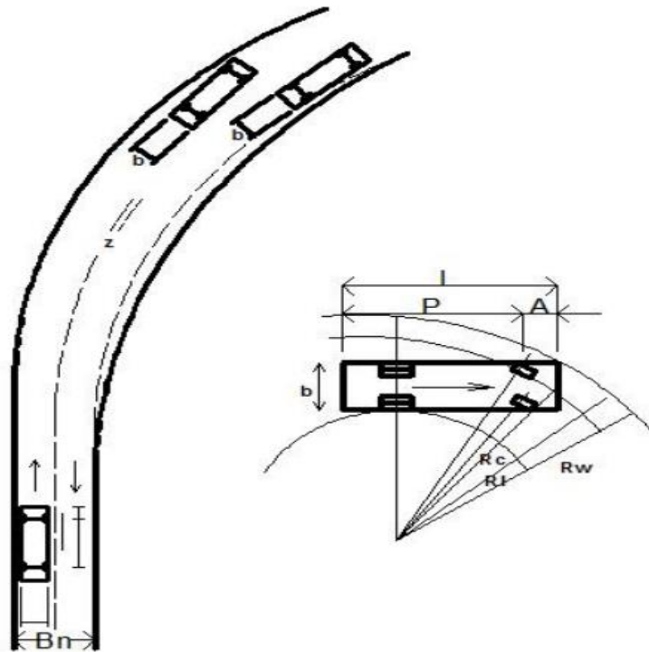
Gambar 2.23 Pelebaran Perkerasan pada Tikungan
