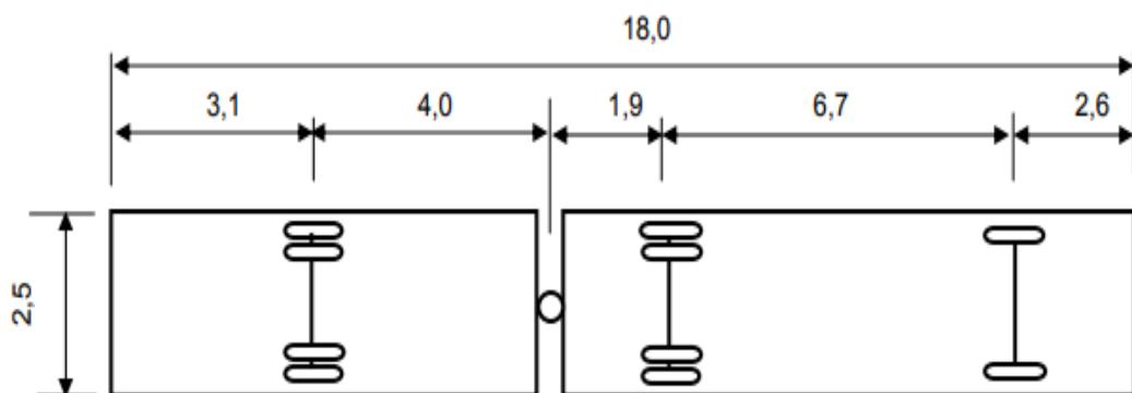
Gambar 2.11 Kendaraan Bus Tempel atau Gandengan (A-BUS)
