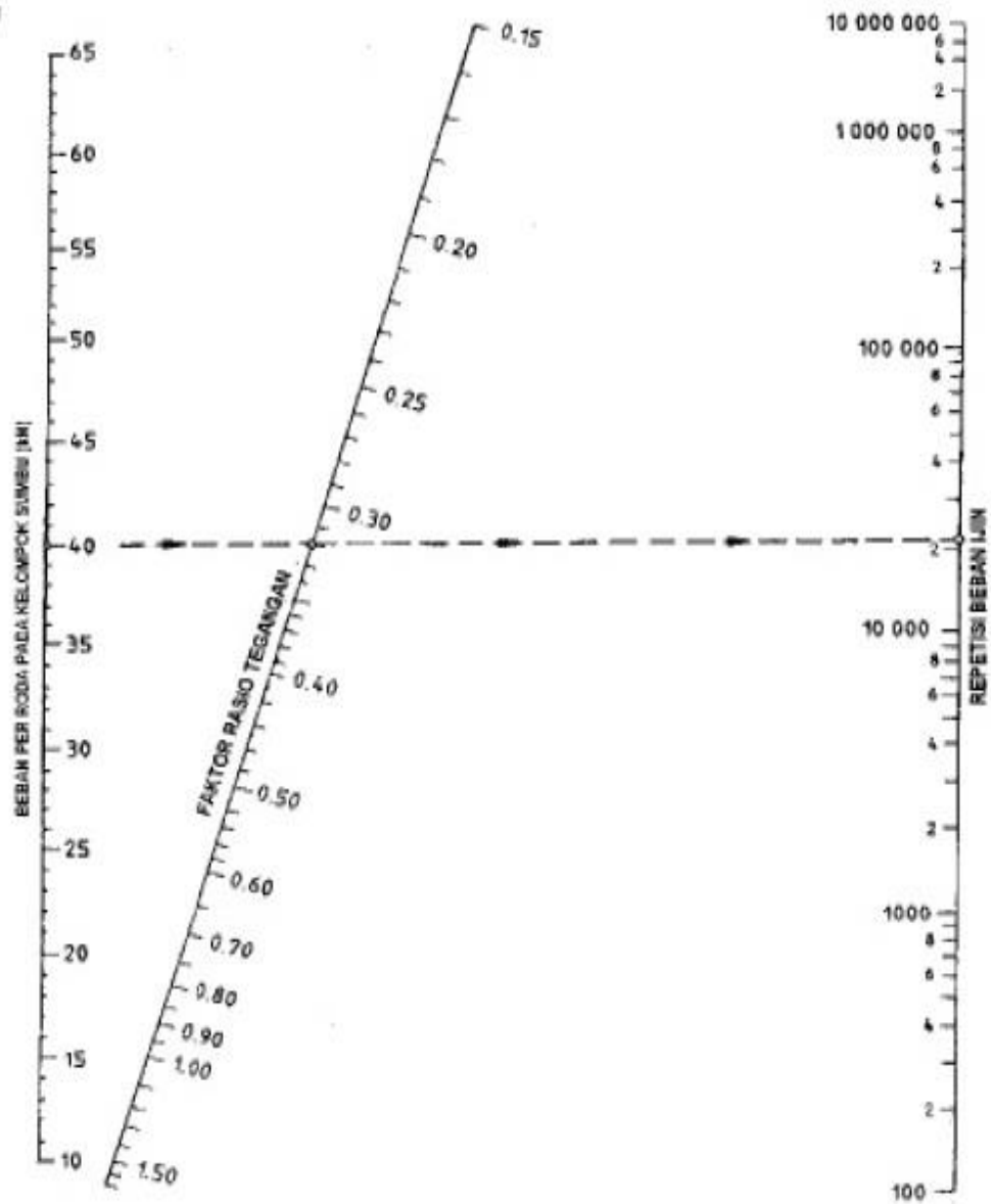
Gambar 2.40 Analisis Fatik dan Beban Repetisi Ijin Berdasarkan Rasio Tegangan, dengan / Tanpa Bahu Beton
