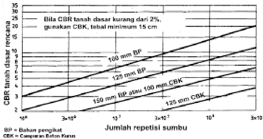
Gambar 2.38 Tebal Pondasi Bawah Minimum untuk Perkerasan Kaku Terhadap Repetisi Sumbu
