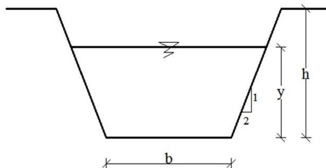
Gambar 2.35 Penampang Saluran Berbentuk Trapesium
