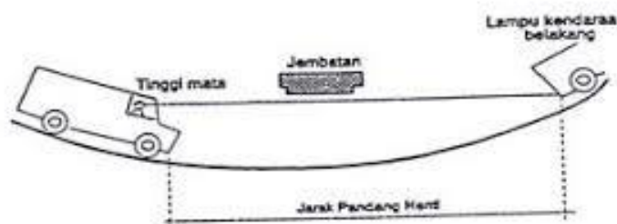
Gambar 2.15 Jarak Pandang Henti pada Lengkung Vertikal Cekung
