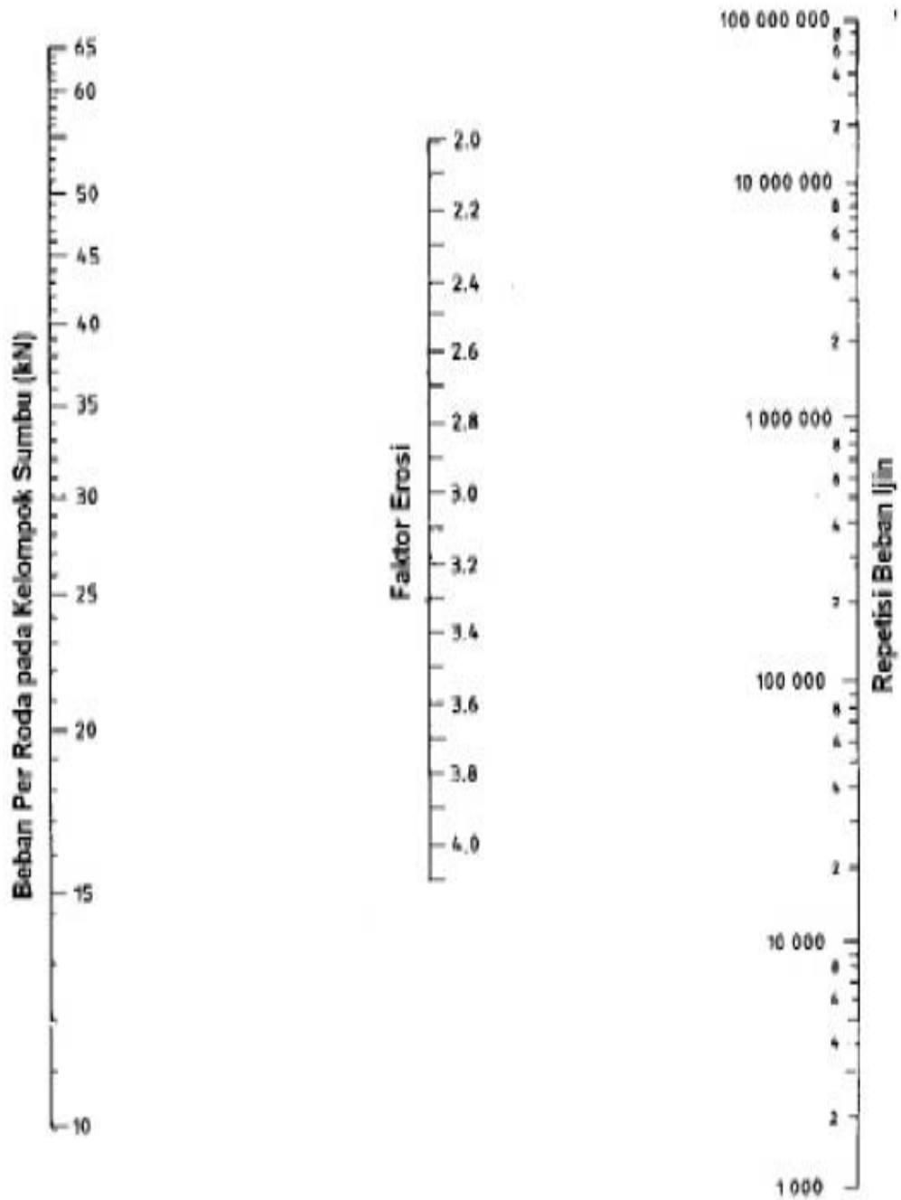
Gambar 2.41 Analisis Erosi dan Jumlah Repetisi Beban Ijin, Berdasarkan Faktor Erosi, Tanpa Bahu Beton
