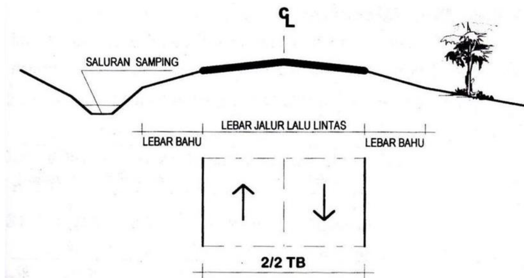
Gambar 2.1 Penampang Melintang Jalan Tanpa Median
