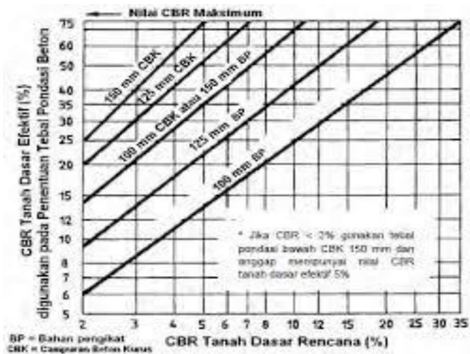
Gambar 2.39 CBR Tanah Dasar Efektif dan Tebal Pondasi Bawah
