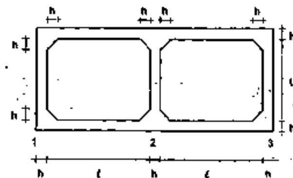
Gambar 2.36 Dimensi Gorong – gorong Persegi
