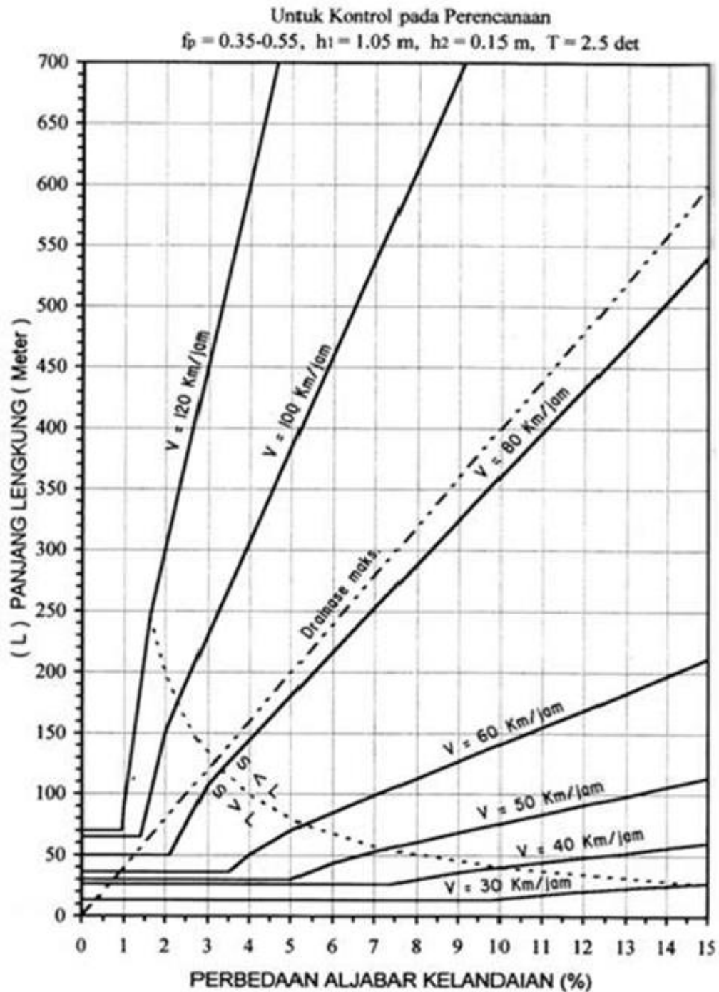
Gambar 2.31 Grafik Panjang Lengkung Vertikal Cembung Berdasarkan Jarak Pandang Henti ( J_h )
