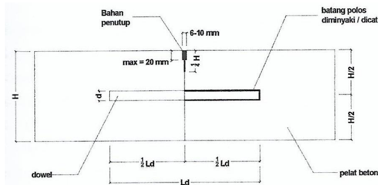
Gambar 2.43 Sambungan Susut Melintang deng Dowel
