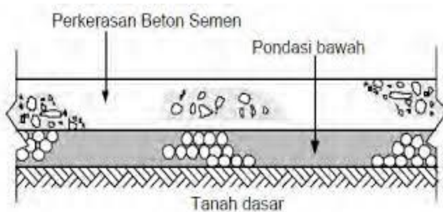
Gambar 2.37 Tipikal Struktur Perkerasan Beton Semen
