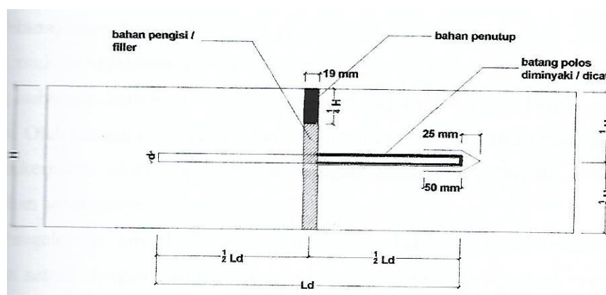
Gambar 2.45 Sambungan Muai dengan Dowel
