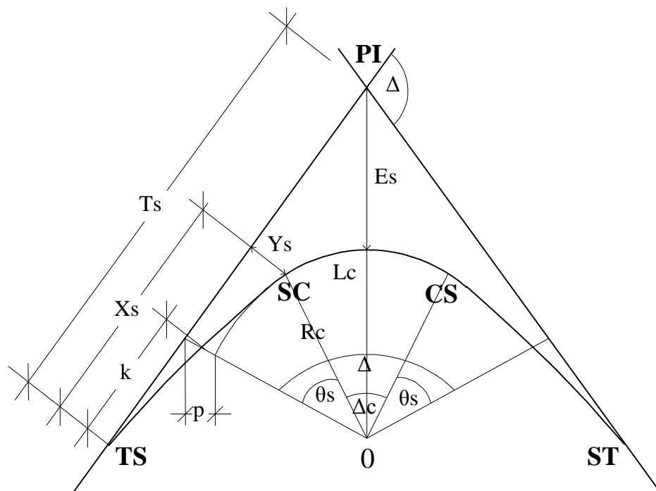
Gambar 2.9 Komponen Spiral-Circle-Spiral
