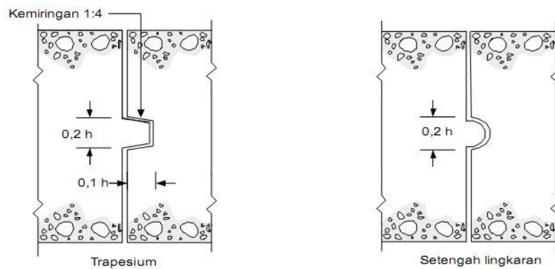
Gambar 2.27 Ukuran Standar Penguncian Sambungan Memanjang
