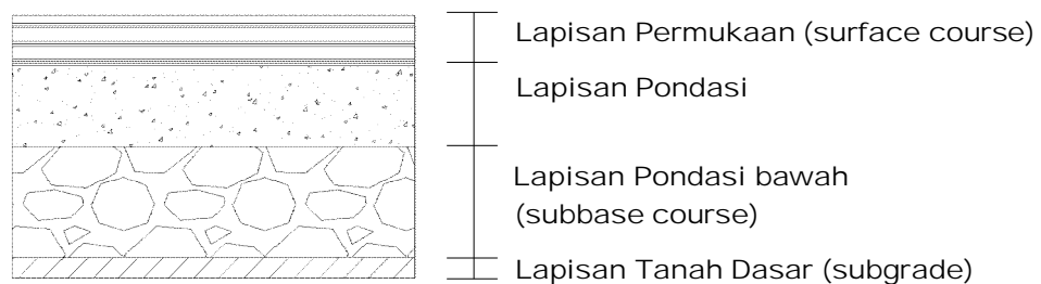
Gambar 2.22 Perkerasan Lentur
