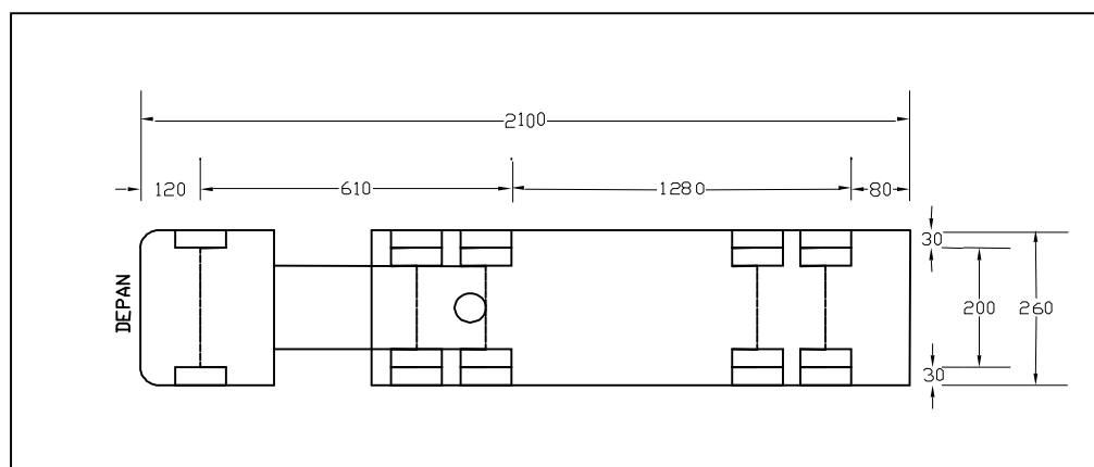
Gambar 2.3 Dimensi Kendaraan Besar
