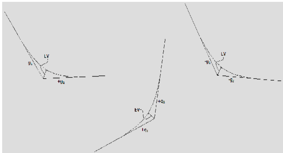
Gambar 2.18 Lengkung Vertikal Cekung
