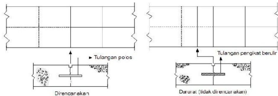
Gambar 2.31 Sambungan Pelaksanaan yang direncanakan dan yang tidak direncanakan untuk pengecoran seluruh lebar perkerasan
