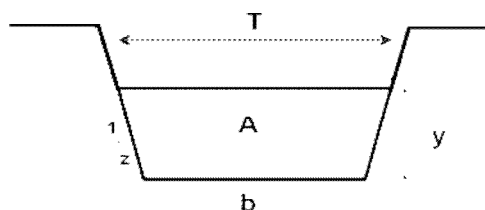
Gambar 2.35 Saluran dengan Bentuk Trapesium
