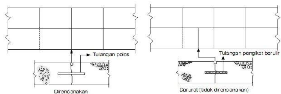
Gambar 2.30 Sambungan Pelaksanaan yang direncanakan dan yang tidak direncanakan untuk pengecoran per lajur
