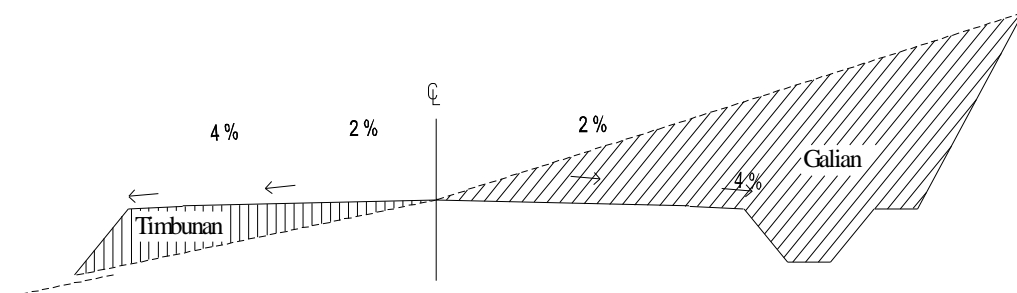
Gambar 2.20 Galian dan Timbunan
