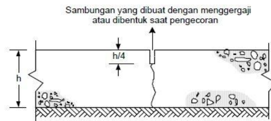
Gambar 2.28 Sambungan Susut Melintang Tanpa Ruji
