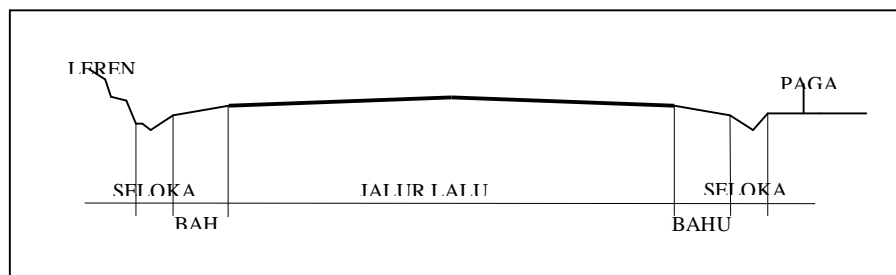
Gambar 2.5 Tipikal Penampang Melintang Jalan
