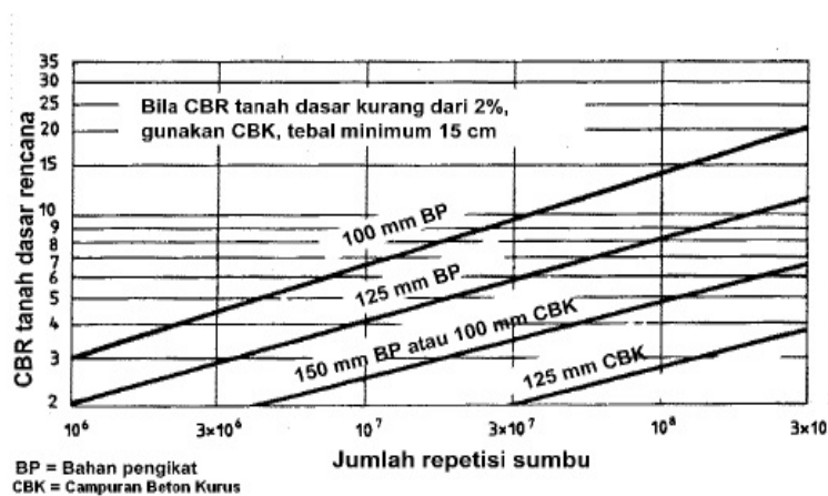
Gambar 2.24 Tebal Pondasi Bawah Minimum untuk Beton Semen
