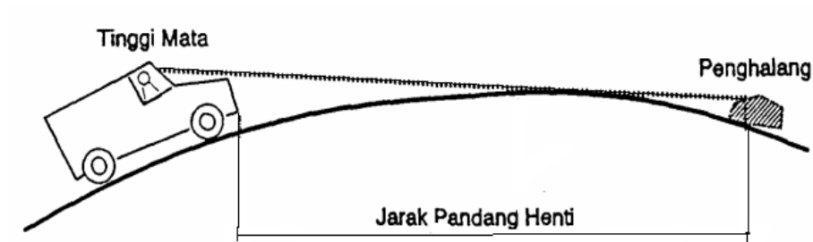
Gambar 2.17 Jarak pandang Lengkung Vertikal Cembung
