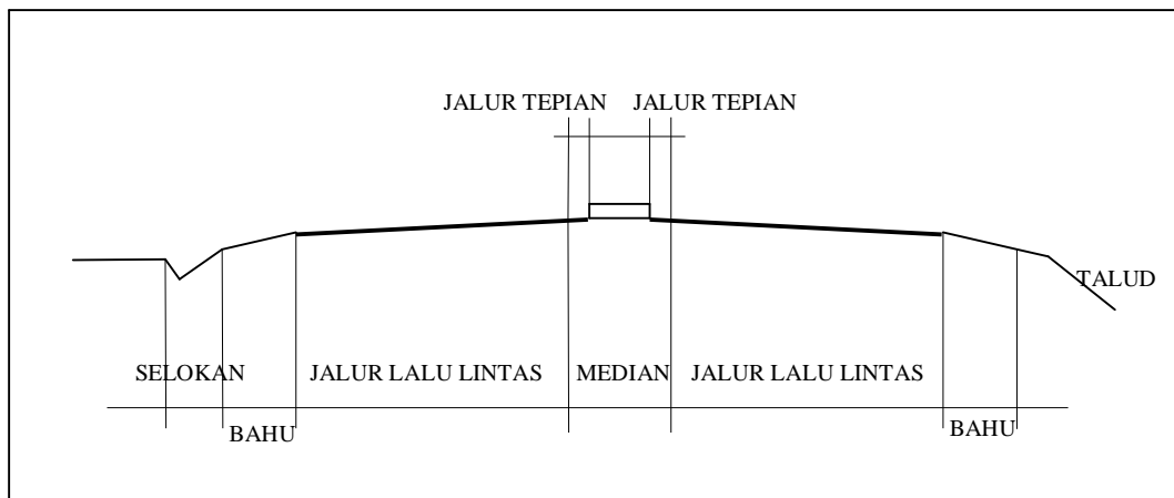
Gambar 2.7 Tipikal Penampang Melintang Jalan yang Dilengkapi Median
