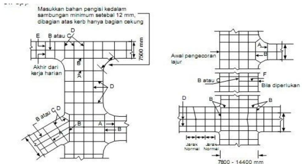
Gambar 2.33 Detail Potongan Melintang Sambungan Perkerasan
