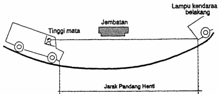
Gambar 2.19 Jarak Pandang Lengkung Vertikal Cekung
