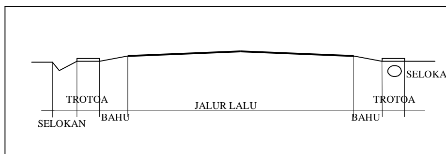
Gambar 2.6 Tipikal Penampang Melintang Jalan yang Dilengkapi Trotoar
