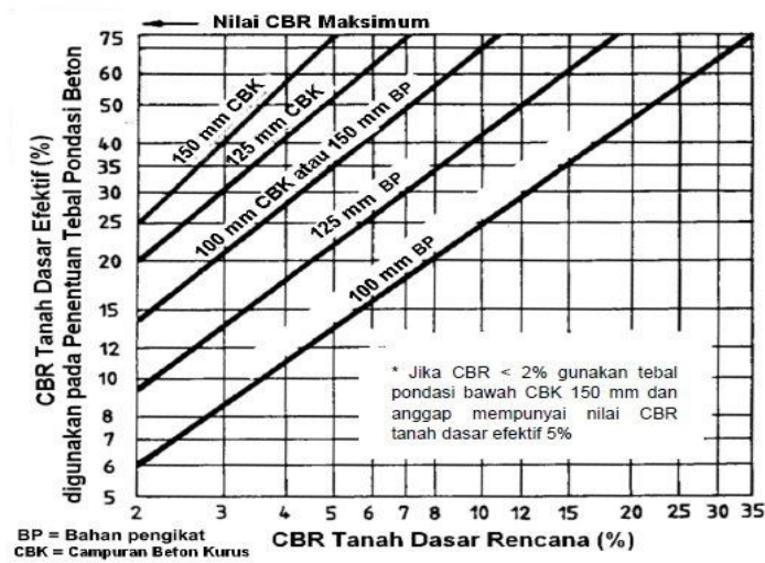
Gambar 2.25 CBR Tanah Dasar Efektif dan Tebal Pondasi Bawah
