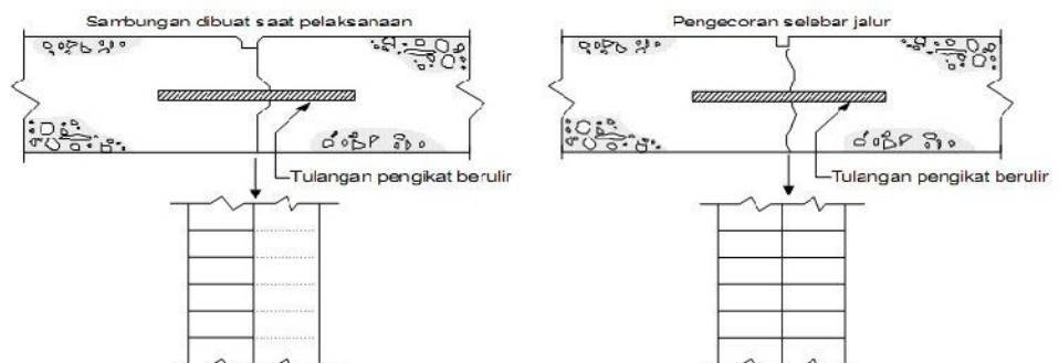
Gambar 2.26 Tipikal Sambungan Memanjang
