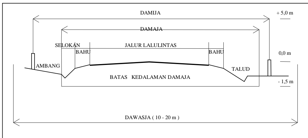
Gambar 2.4 Damaja, Damija dan Dawasja di lingkungan jalan antar kota
