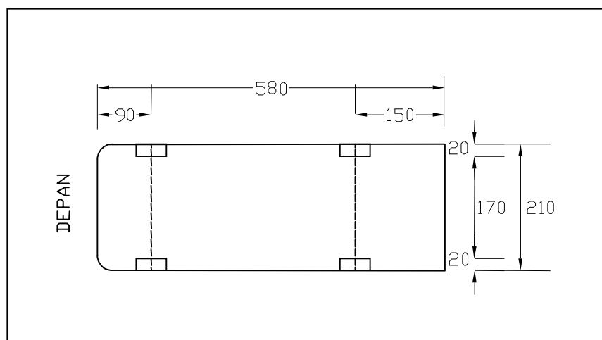
Gambar 2.1 Dimensi Kendaraan Kecil
