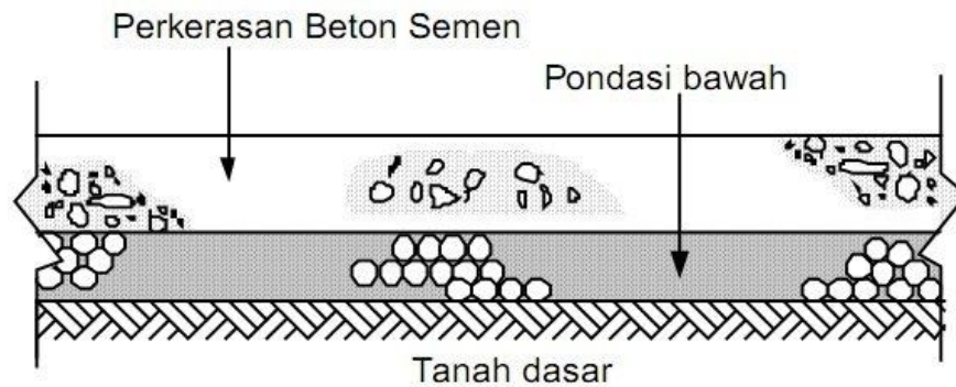
Gambar 2.23 Susunan Lapisan Perkerasan Kaku
