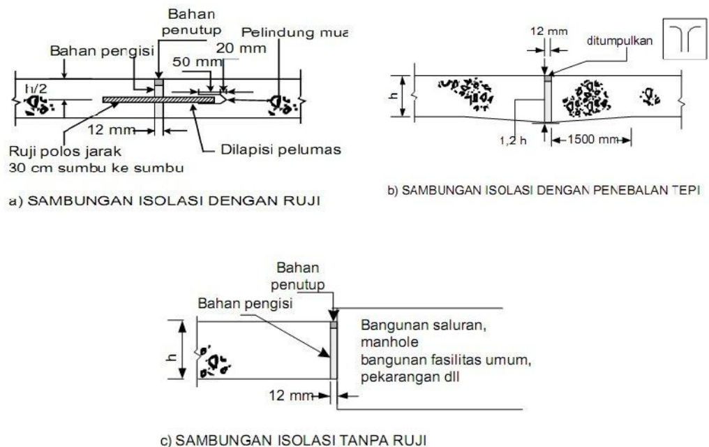
Gambar 2.32 Sambungan Isolasi
