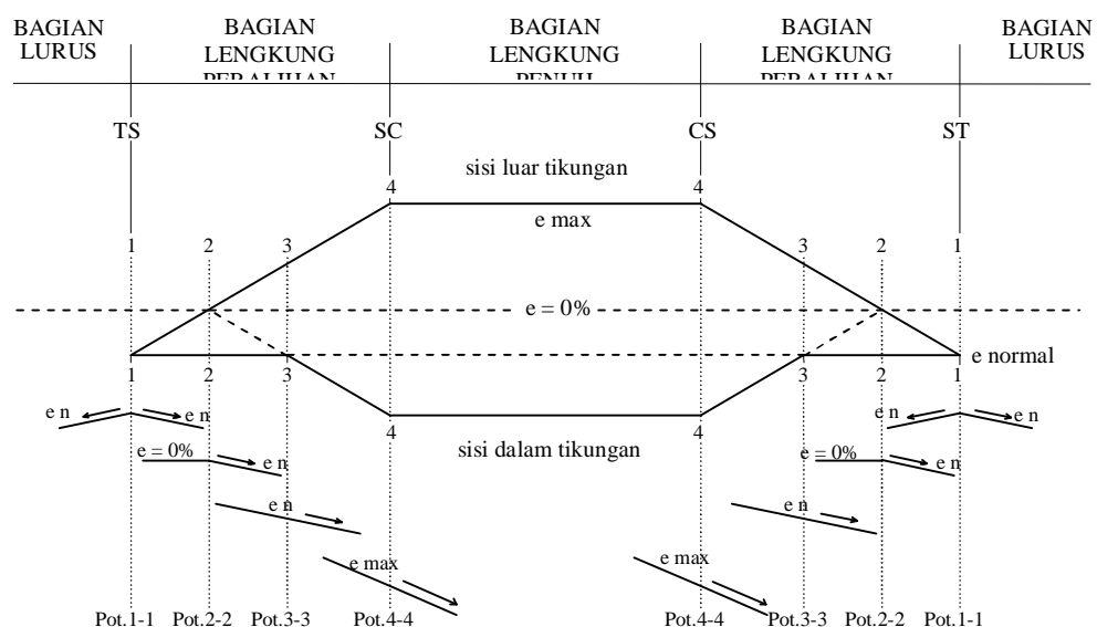
Gambar 2.11 Metoda Pencapaian Superelevasi pada Tikungan Spiral – Circle – Spiral (contoh untuk tikungan ke kanan)
