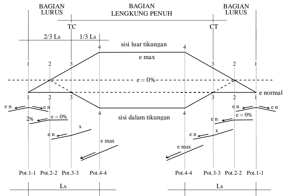
Gambar 2.12 Metoda Pencapaian Superelevasi pada Tikungan Full Circle (contoh untuk tikungan ke kiri)
