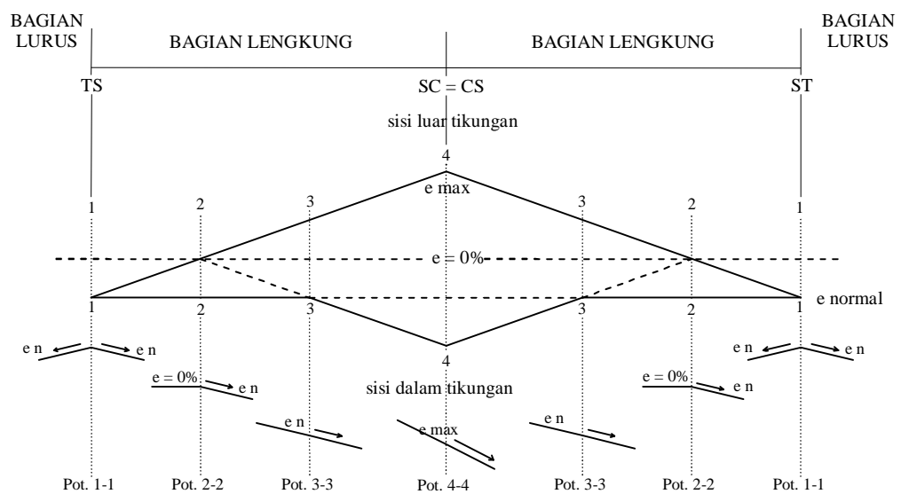
Gambar 2.13 Metoda Pencapaian Superelevasi pada Tikungan Spiral – Spiral (contoh untuk tikungan ke kanan)
