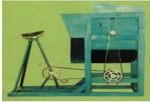
Gambar 2.3 Alat Pemipil Jagung Model Ban
