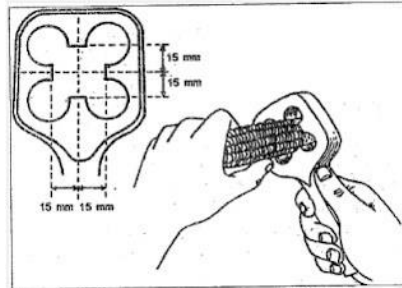
Gambar 2.1 Alat Pemipil Jagung Model TPI
