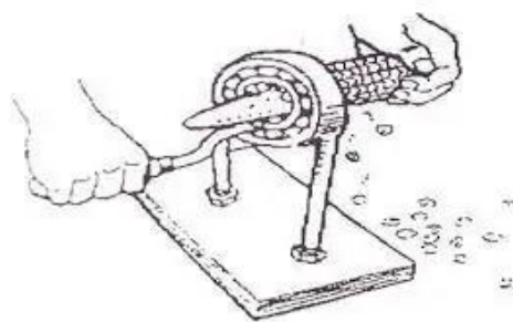
Gambar 2.2 Alat Pemipil Jagung Model Langer
