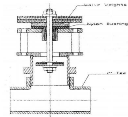
Gambar 2.6 Desain Klep Limbah
