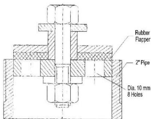
Gambar 2.7 Desain Klep Penghantar
