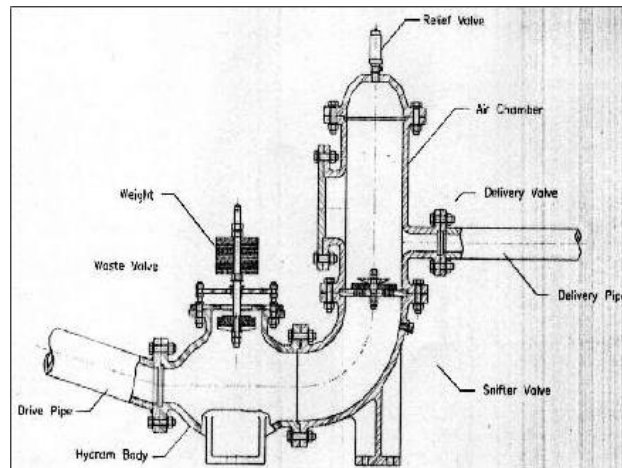
Gambar 2.5 Desain Pompa Hidram
