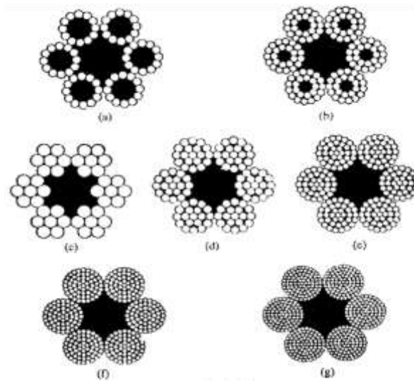
Gambar 2.21 Jenis-jenis lilitan kawat sling (megajaya 2020)
