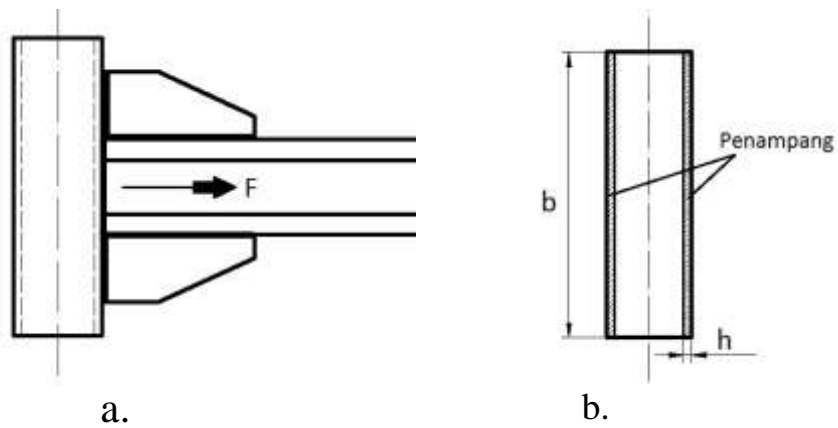
Gambar 2.27 posisi Pilar Putar mendapat beban tarik (a) dan (b) posisi penampang Pilar Putar (eprints 2020)
