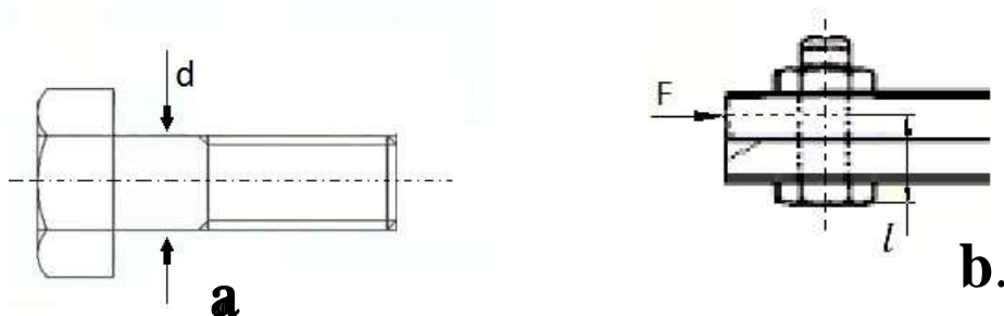
Gambar 2.28 Diameter baut (a) dan posisi baut mendapat beban (b) (eprints 2019)
