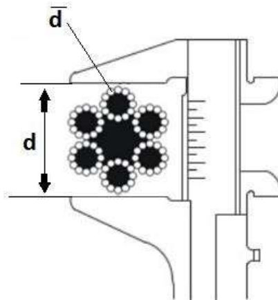
Gambar 2.31 Mencari diameter sling (kpssteel 2020)
