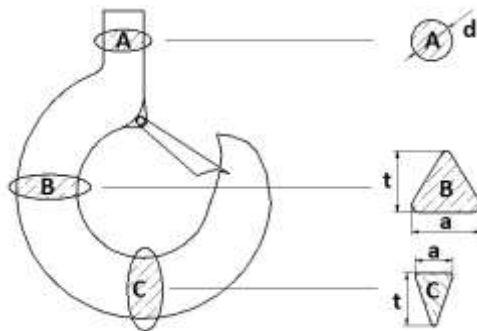
Gambar 2.32 Titik beban hook (enzdooc 2013)
