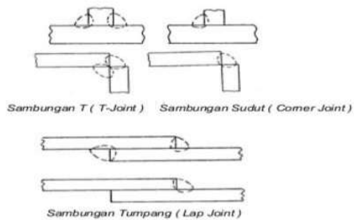
Gambar 2.12 Jenis-jenis Pengelasan (Penjelasn 2020)
