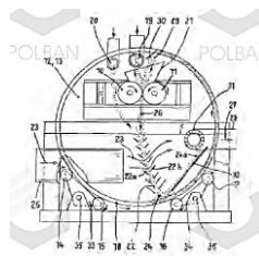
Gambar 2.1 Roller Mill (Mardiansyah, 2012)
