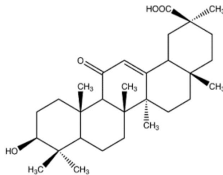
Gambar 2.8 Struktur Senyawa Triterpenoid (illing,2017)
