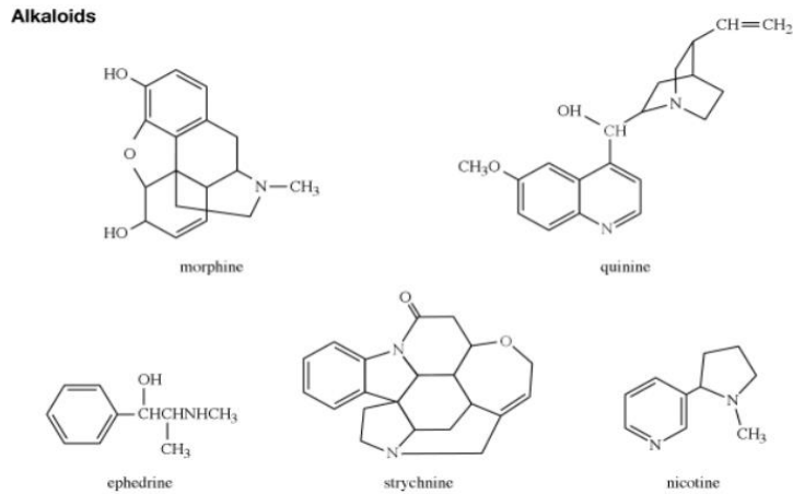
Gambar 2.4 Struktur senyawa alkhaldoid (Noer, Pratiwi Gresinta, 2013)
