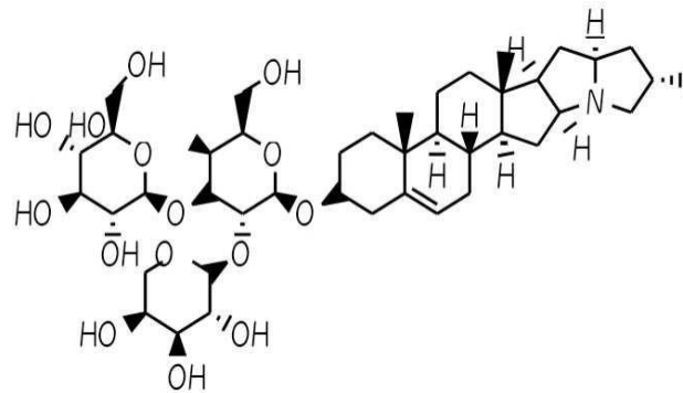
Gambar 2.5 Struktur Senyawa Saponin (illing,2017)
