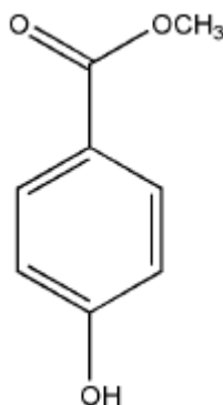
Gambar 2.13 Struktur Kimia Metil Paraben
