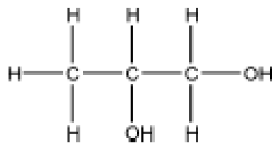
Gambar 2.11 Struktur Kimia Propilen Glikol
