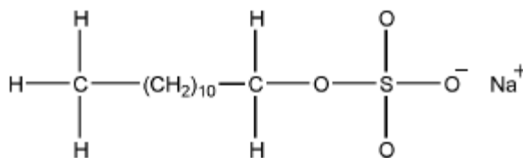
Gambar 2.9 Struktur kimia sodium lauryl sulfat
