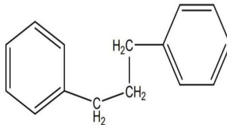
Gambar 2.6 Struktur Senyawa Flavanoid (Noer,Pratiwi,Gresinta,2013)
