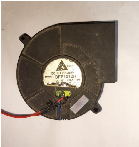
Gambar L3.11 Mini Blower
