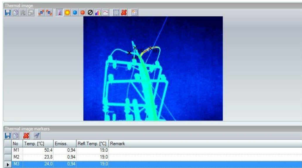
Gambar 3.1 Thermal Image Hasil Temuan Hot Spot
