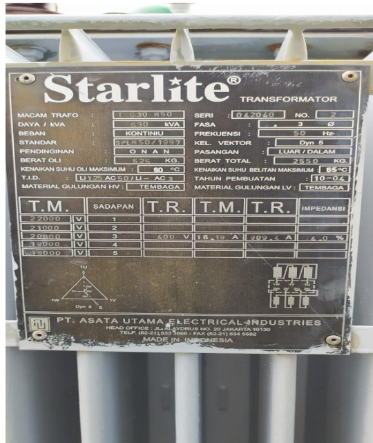
Gambar Nameplat pada Transformator Daya PS Unit 3
