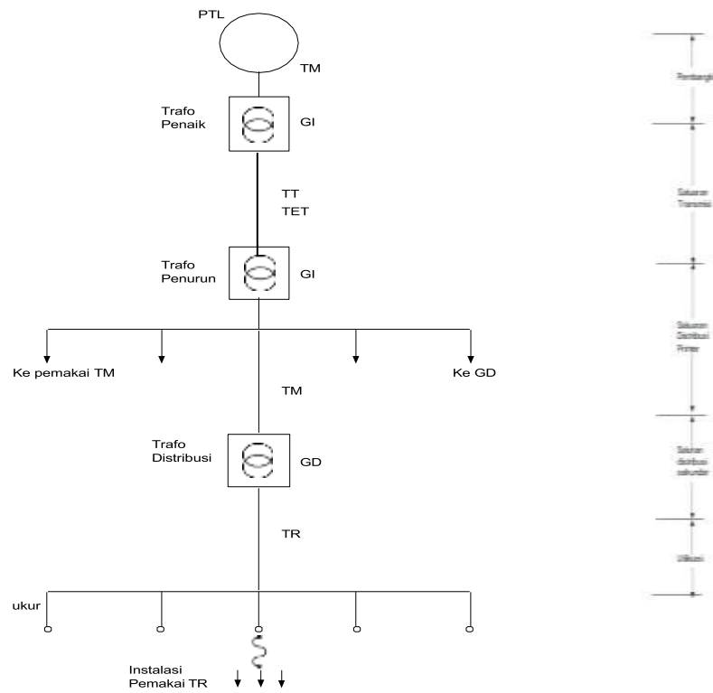
Gambar 2.1. Diagram satu garis sistem tenaga listrik
