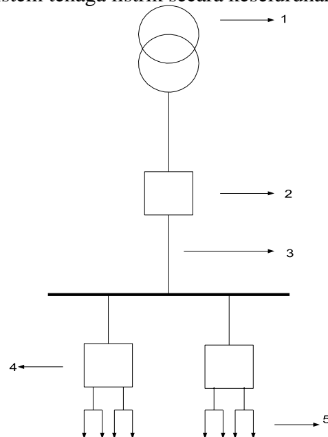
Gambar 2.2 Bagian-bagian sistem distribusi primer
