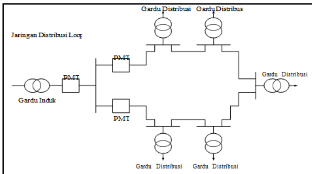
Gambar 2.4 Konfigurasi jaringan distribusi tipe loop
