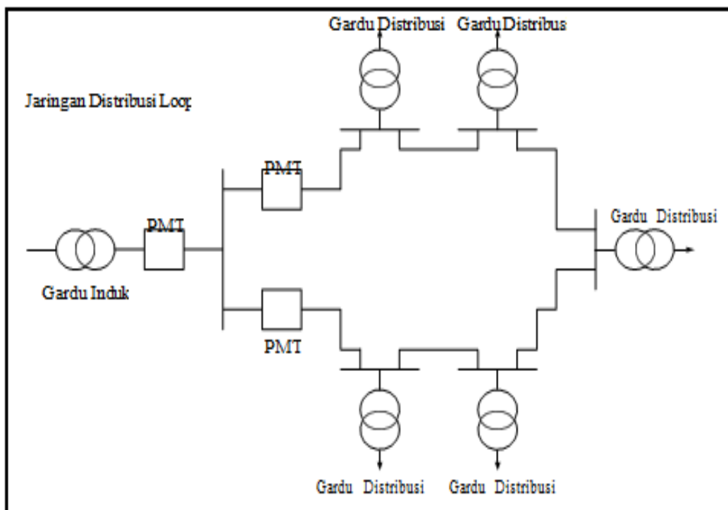
Gambar 2.5 Konfigurasi jaringan distribusi tipe ring
