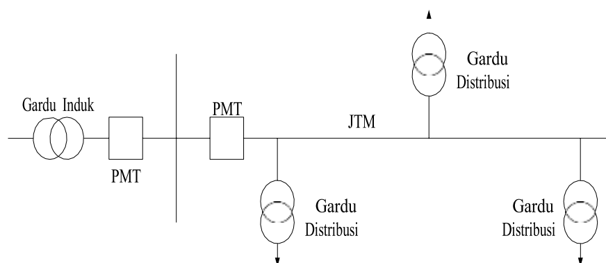
Gambar 2.3 Konfigurasi jaringan distribusi radial
