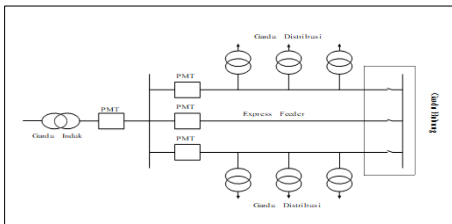
Gambar 2.6 Konfigurasi jaringan spindel
