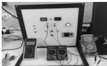
Gambar 2. Peralatan pengukuran potensial.
