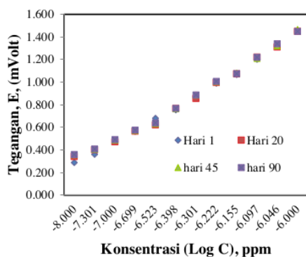
Gambar 7. Grafik stabilitas sensor simazin
