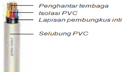
Gambar 2. 9 Konstruksi Kabel NYM
