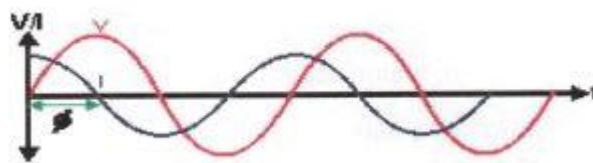
Gambar 2. 34 Gelombang Faktor Daya Mendahului
