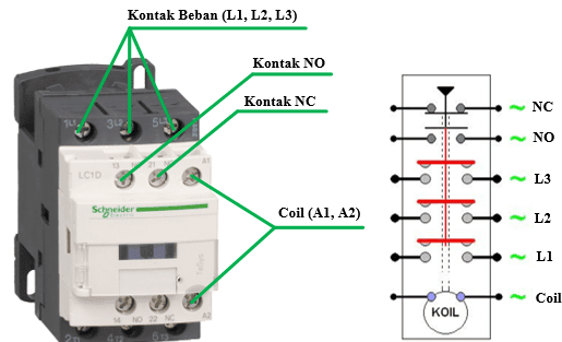
Gambar 2. 5 Kontaktor
