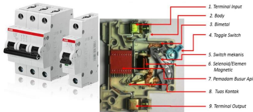
Gambar 2. 4 MCB 1 Fasa dan MCB 3 Fasa
