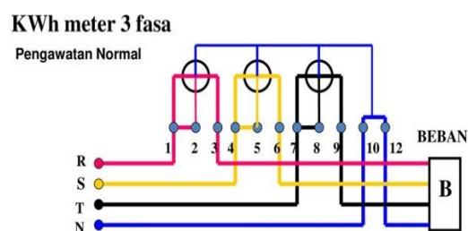
Gambar 2. 2 KWH Meter 3 Fasa
