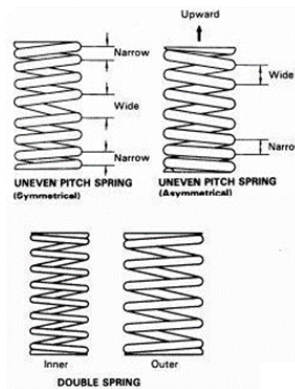
Gambar 2.11 Pegas Katup (Iksotomotif, 2022)
