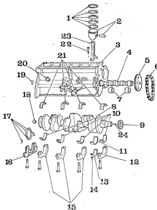
Gambar 2.1 Konstruksi Block Cylinder (Lenterahidup, 2021)
