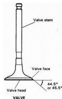
Gambar 2.10 Kepala Katup dan Batang Katup (lksotomotif, 2022)
