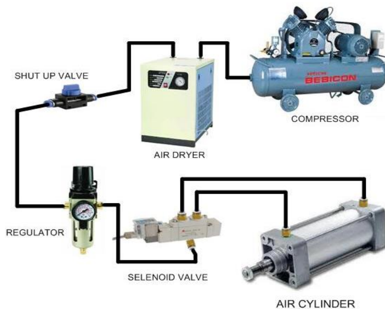
Gambar 2.14 Sistem Pneumatik (trikuenidesain, 2022)
