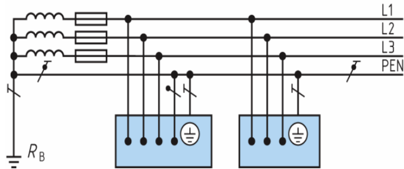
Gambar 2. 7 Saluran Tanah dan Netral disatukan (TN-C)
