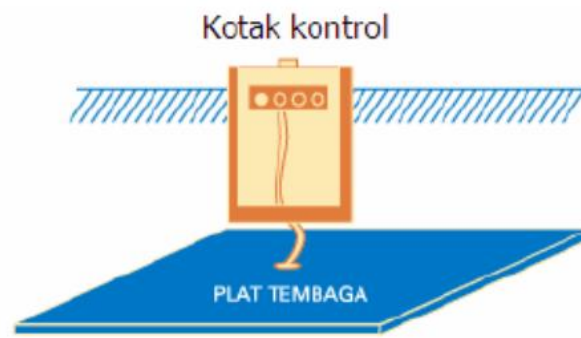
Gambar 2. 15 Elektroda Pelat
