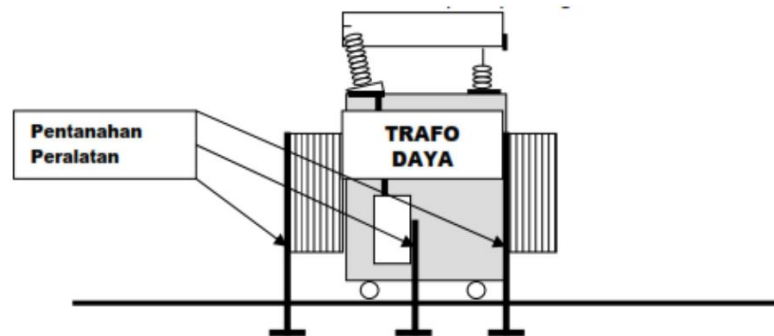
Gambar 2. 12 Pemasangan Pentanahan Peralatan
