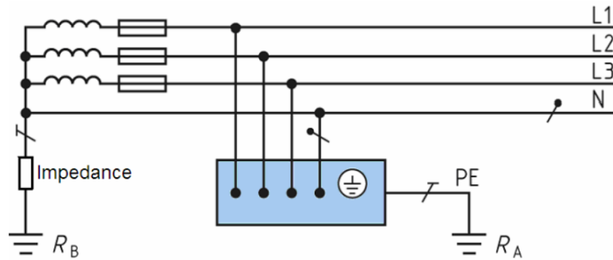
Gambar 2. 11 Saluran Tanah melalui Impedansi (IT)
