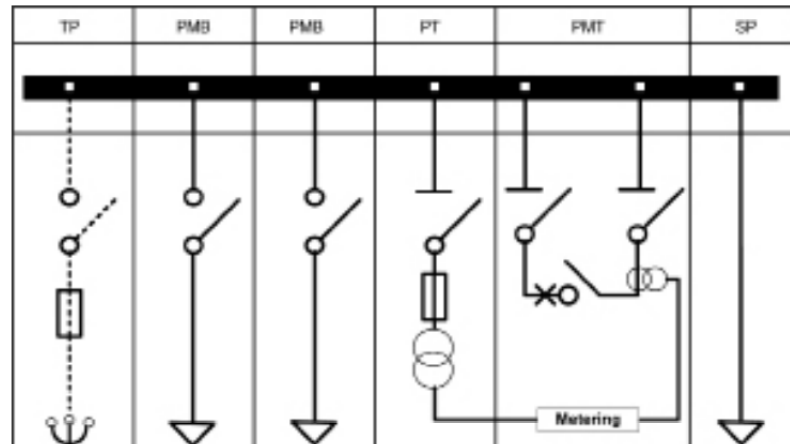
Gambar 2. 22 Bagan satu garis Gardu Pelanggan Khusus
