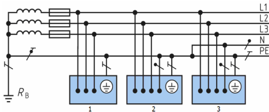
Gambar 2. 8 Saluran Tanah dan Netral disatukan pada sebagian sistem (TN-C-S)
