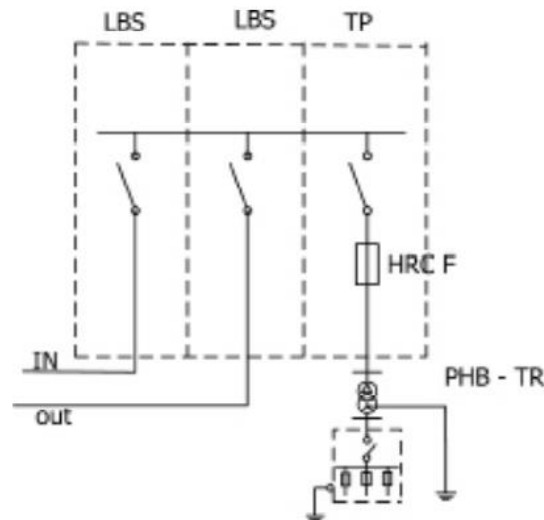
Gambar 2. 21 Bagan satu garis Konfigurasi \pi section Gardu Pelanggan Umum
