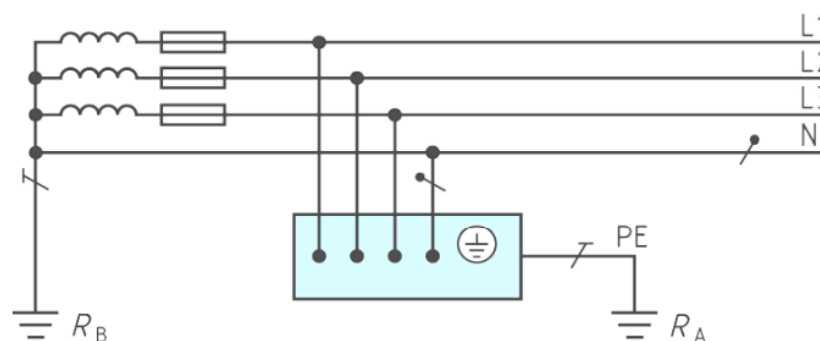
Gambar 2. 10 Saluran Tanah dan Saluran Bagian Sistem Terpisah (TT)
