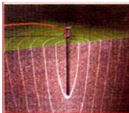
Gambar 2. 6 Batang Pentanahan dan Lingkaran Pengaruhnya. [6]
