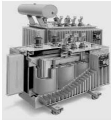
Gambar 2. 23 Transformator Distribusi Fasa 3 yang dibelah
