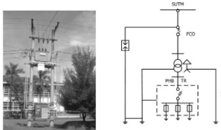
Gambar 2. 16 Gardu Tiang Portal dan Bagan Satu Garis
