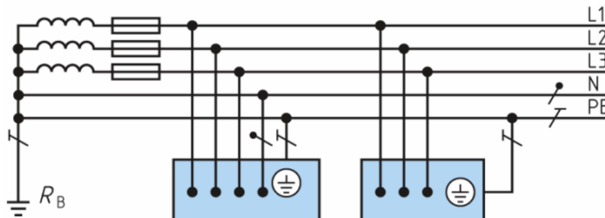
Gambar 2. 9 Saluran dan Netral dipisah (TN-S)
