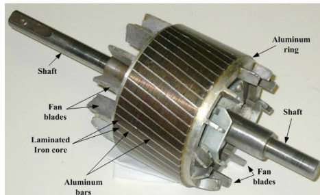
Gambar 2.21 Rotor Sangkar
