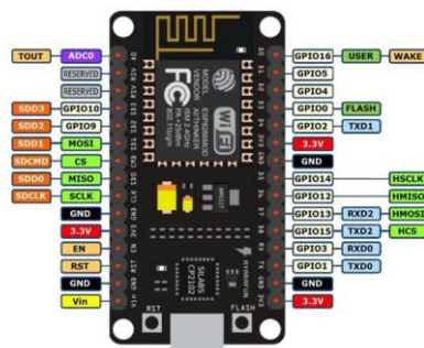
Gambar 2.2 NodeMCU ESP8266 Dan Skema Pin
