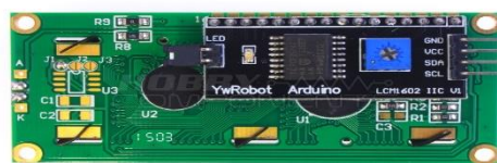
Gambar 2.6 I2C LCD 16 x 2 Karakter
