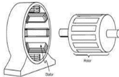
Gambar 2.17 Konstruksi Motor Induksi Satu Fasa
