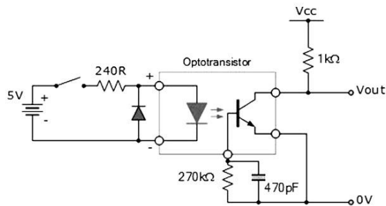
Gambar 2.4 Rangkaian Modul Relay
