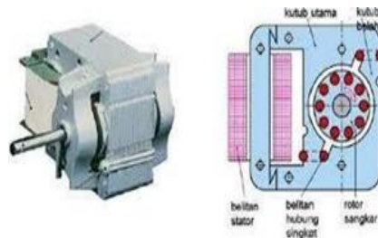
Gambar 2.23 Bentuk Fisik Motor Shaded Pole
