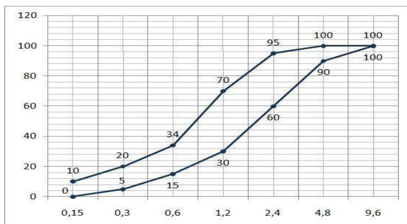
Gambar 2.2 Gradasi Pasir Kasar (Gradasi zone 1 berdasar SNI-03-2834-2000)
