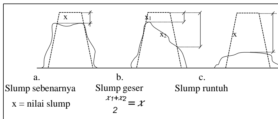
Gambar 2.9 Jenis-jenis Slump
