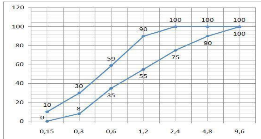
Gambar 2.3 Gradasi Pasir Sedang (Gradasi zone 2 berdasar SNI-03-2834-2000)
