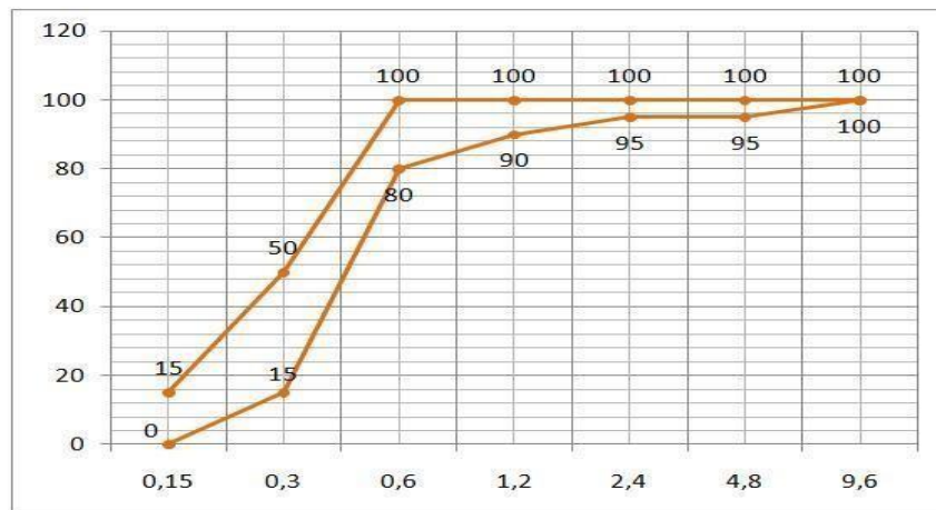
Gambar 2.5 Gradasi Pasir Halus (Gradasi Zone 4 berdasar SNI-03-2834-2000)
