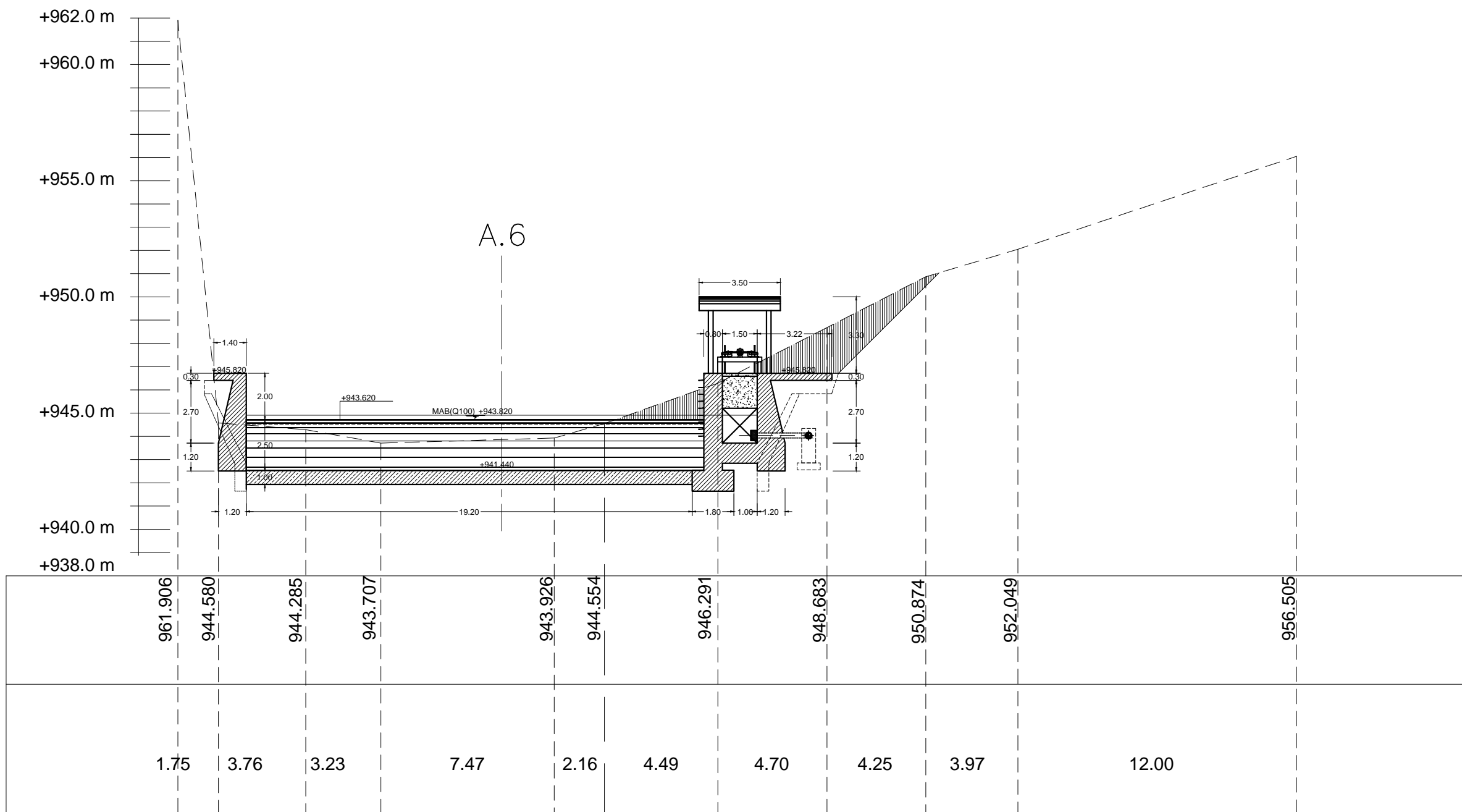
Potongan 4 - 4 Skala 1 : 100
