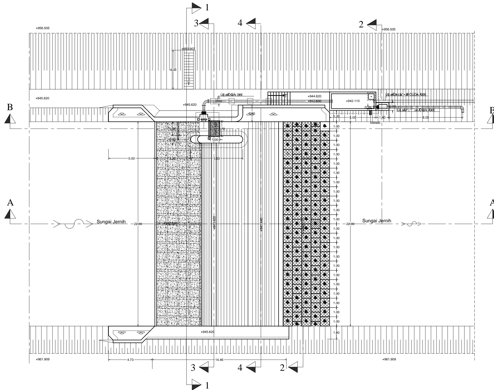
DENAH Skala 1 : 100
