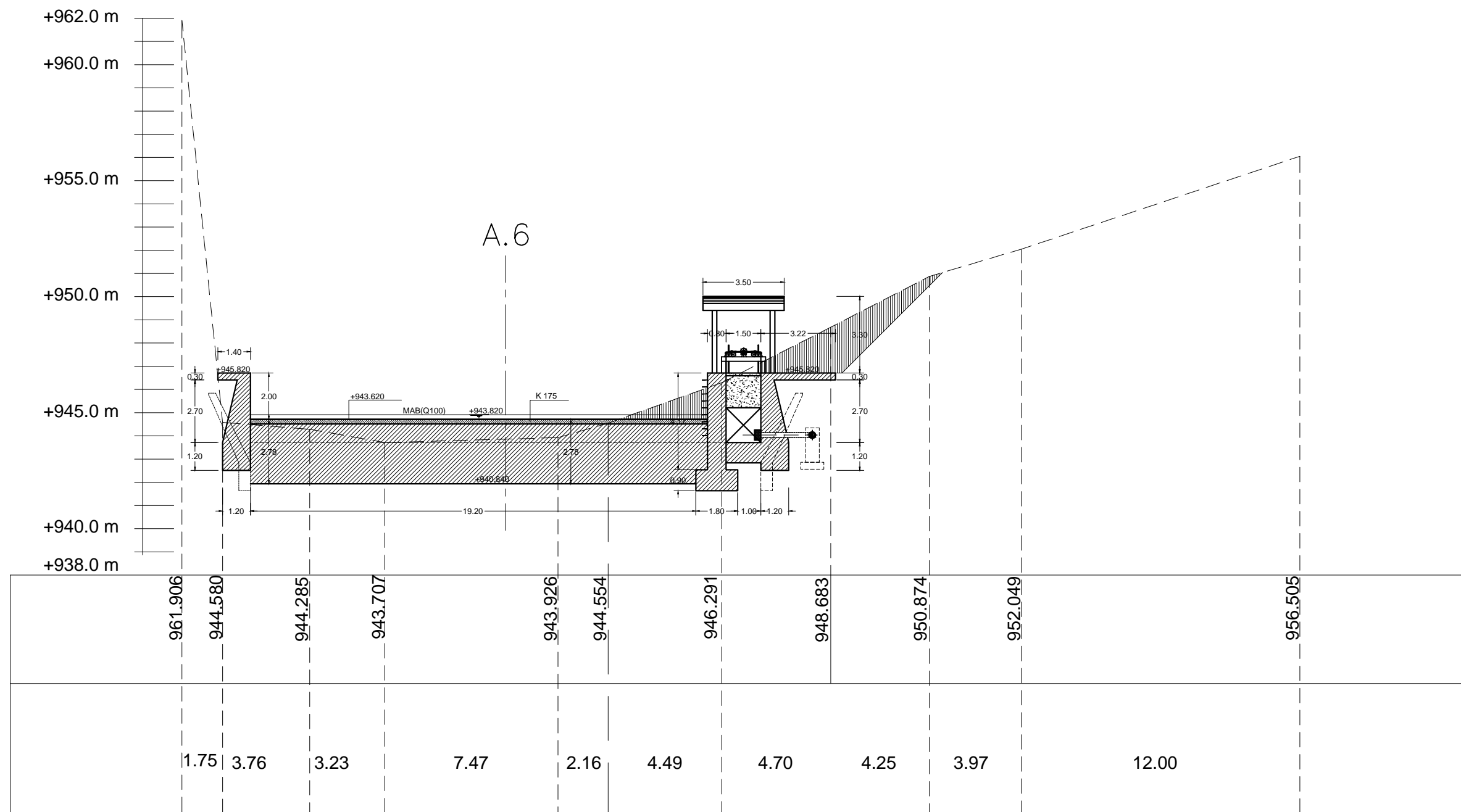
Potongan 3 - 3
