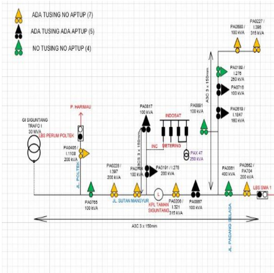
Single Line Diagram Penyulang Banteng
