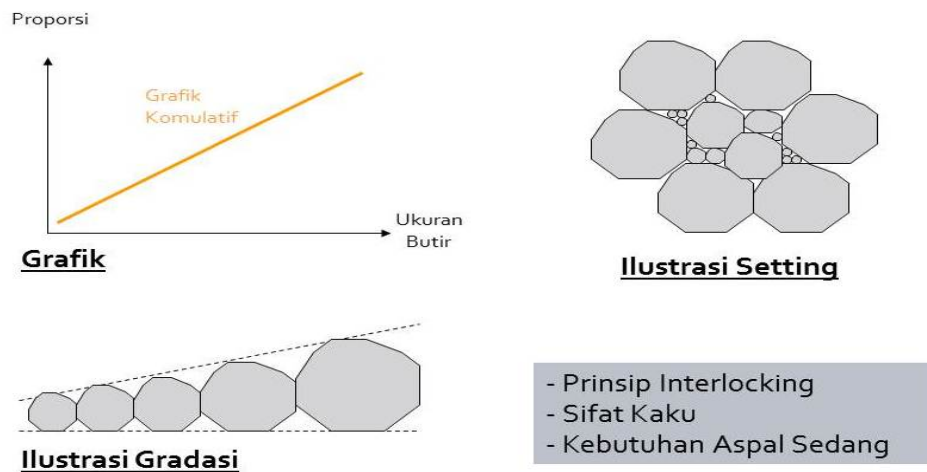
Gambar 2.4 Ilustrasi Gradasi Menerus
