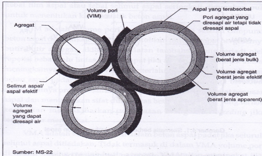
Gambar 2.5 Rongga Dalam Campuran
