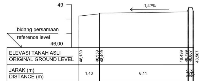
STA 1+750
