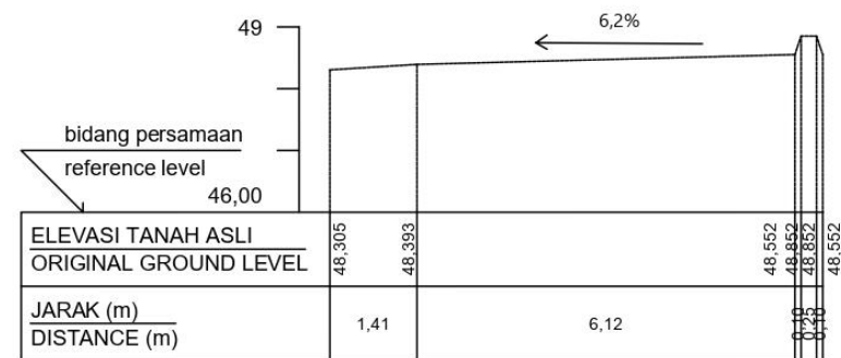
STA 1+000
