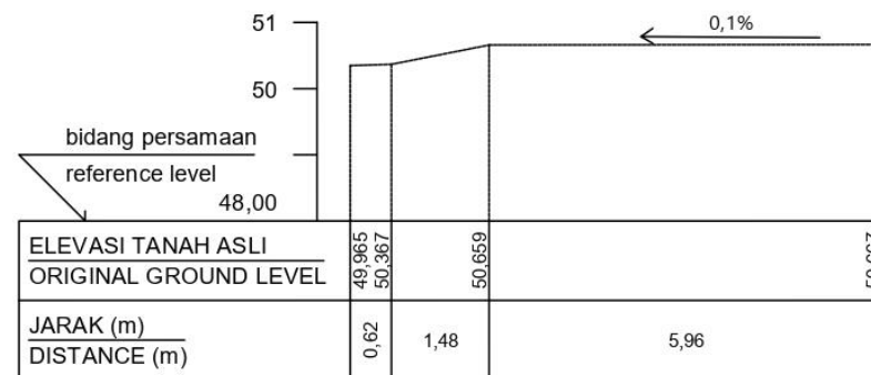
STA 0+200
