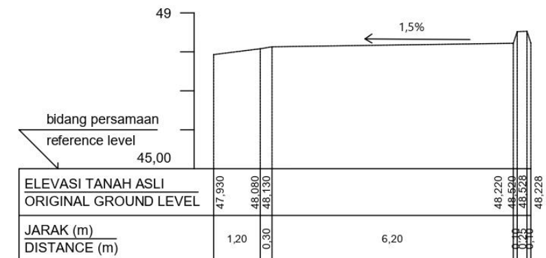
STA 1+250
