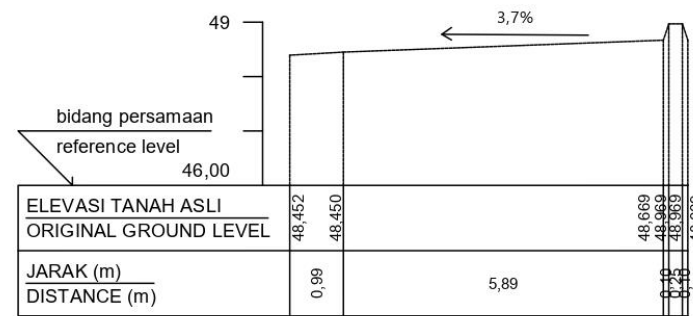
STA 0+900
