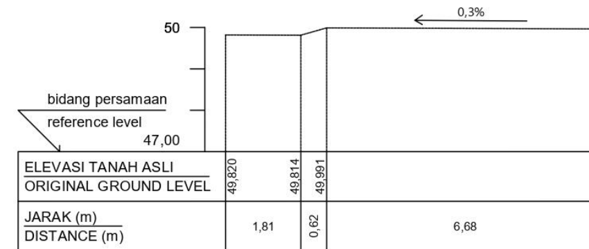
STA 0+125
