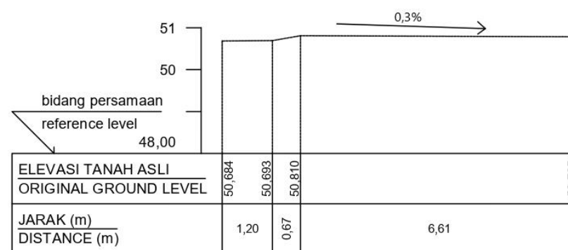
STA 0+250
