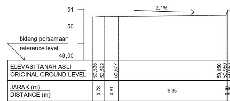
STA 0+375
