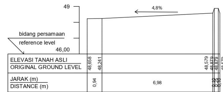
STA 0+925
