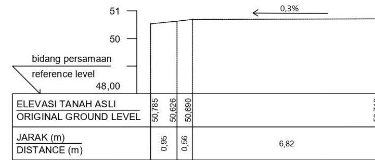
STA 0+325
