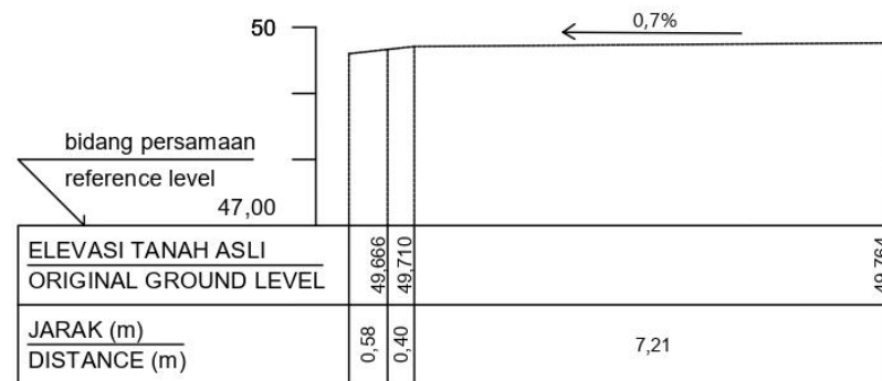
STA 0+100
