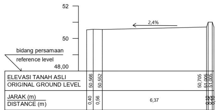
STA 0+350
