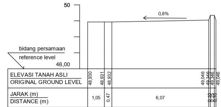
STA 0+625
