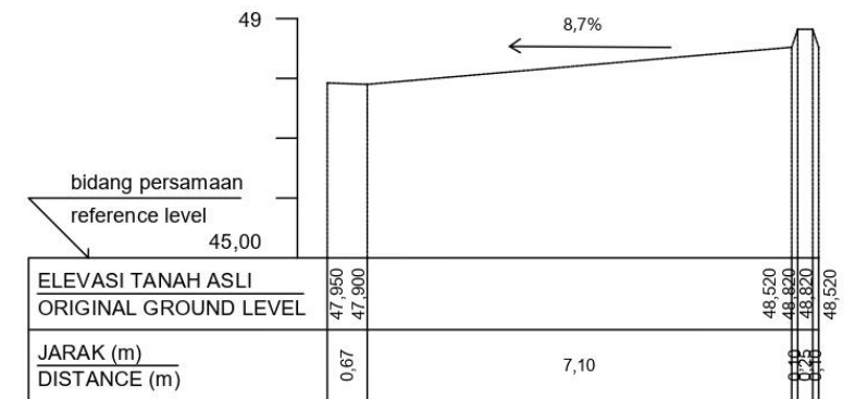
STA 0+775
