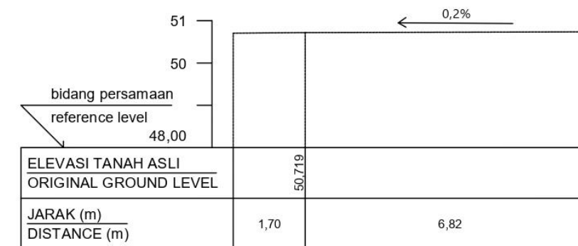
STA 0+225
