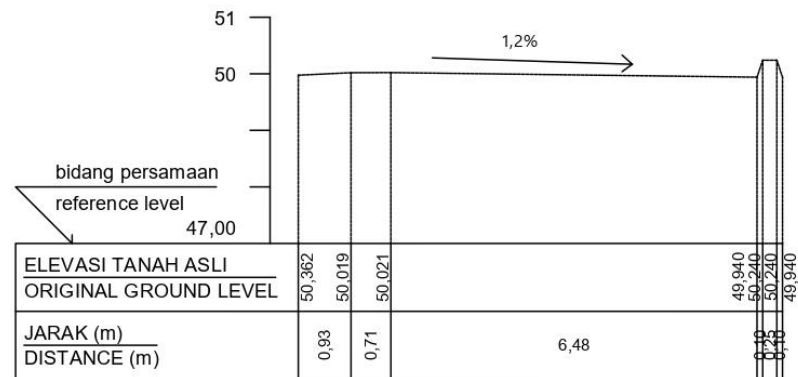
STA 0+550
