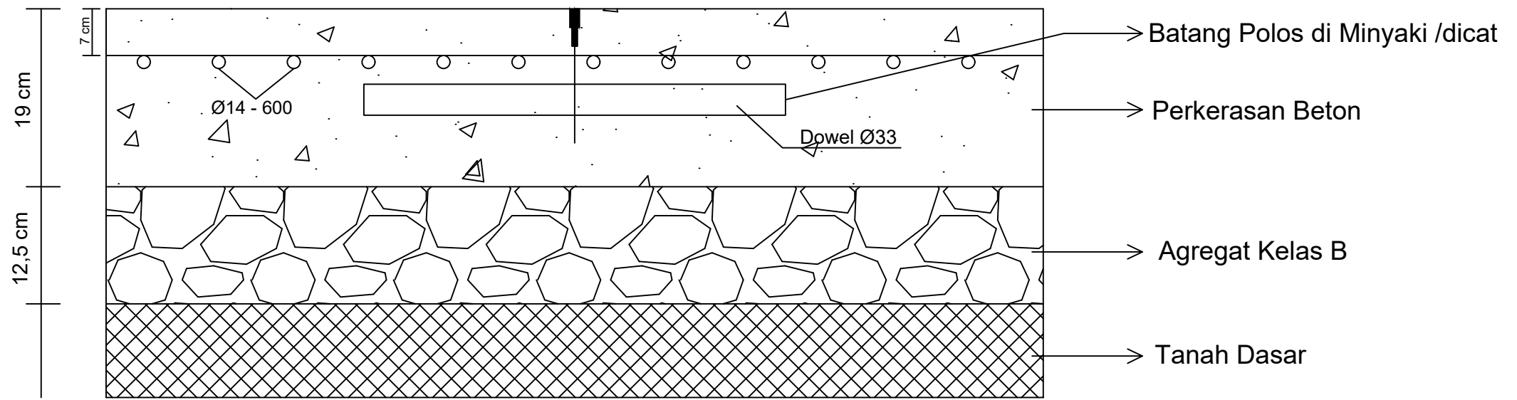
Gambar Penulangan Melintang dan Sambungan Dowel
