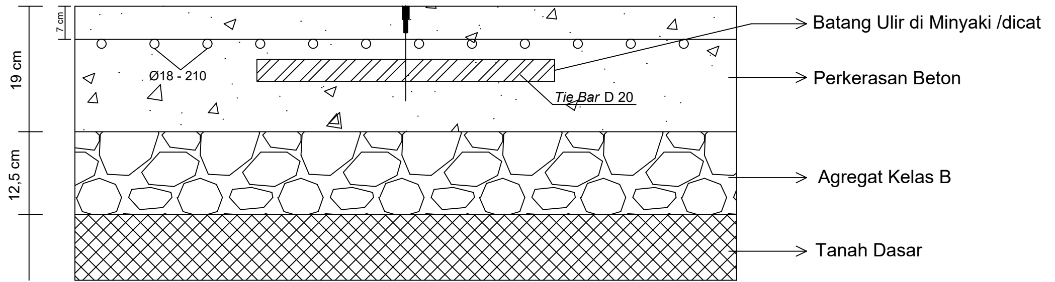
Gambar Penulangan Memanjang dan Sambungan Tie bar
