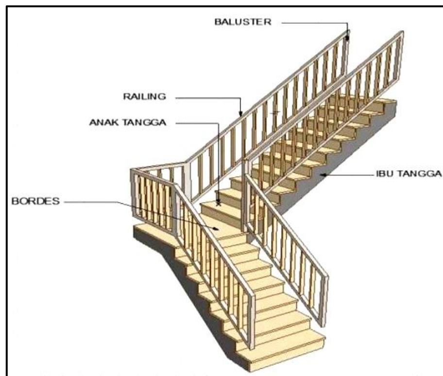
Gambar 2.6 Bagian-bagian tangga
