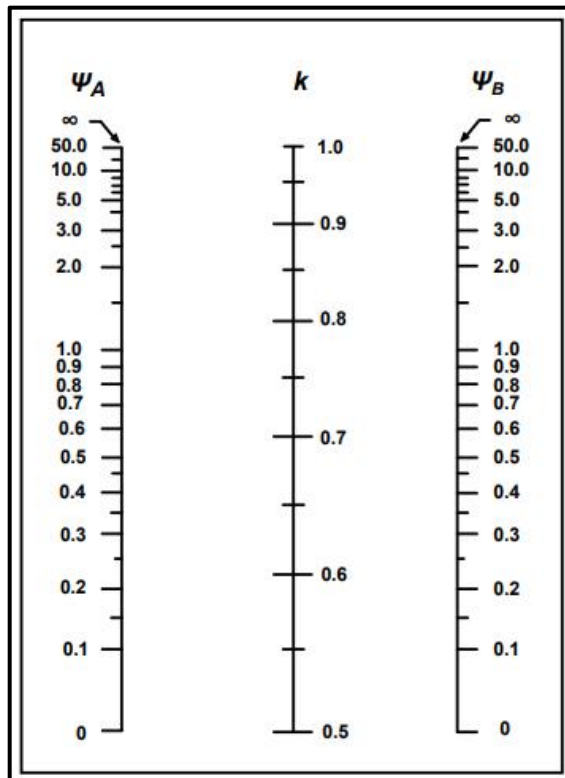
Gambar 2. 19 Grafik Komponen Struktur tak Bergoyang
