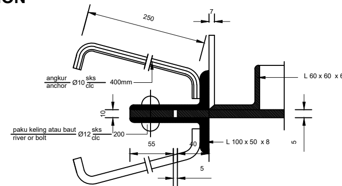
POTONGAN SECTION
