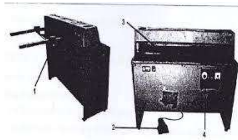
Gambar 2.1 Mesin guillotine (Mudirianto, 2016)
