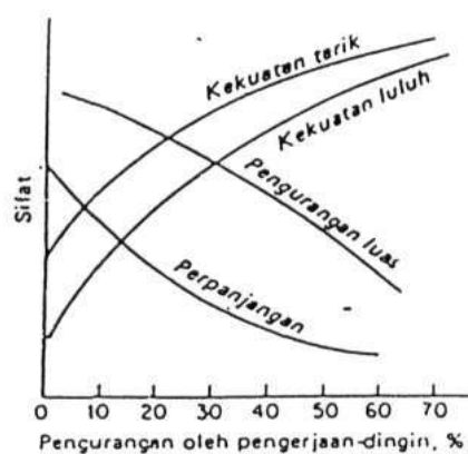
Gambar 2.8 Perlakuan bending oleh pengerjaan dingin (Fazri, 2023)
