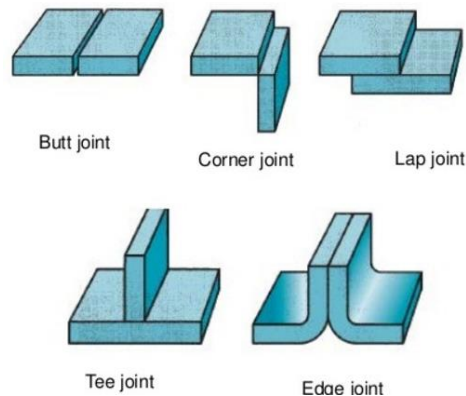
Gambar 2.1 Sambungan Las (Fazri, 2023)
