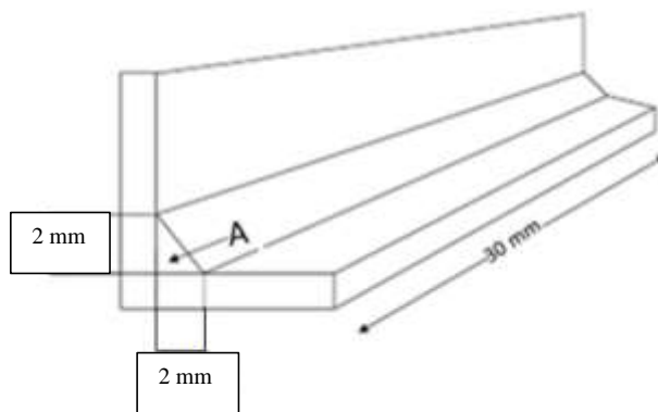
Gambar 2.11 Sambungan Las
