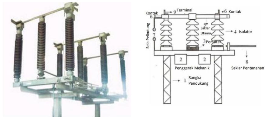
Gambar 2.1 Pemisah (PMS)
