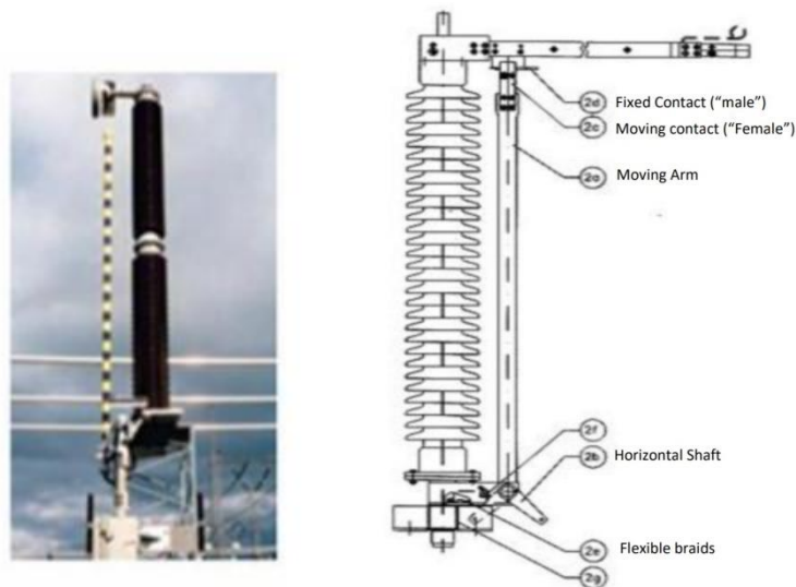
Gambar 2.6 Pisau Pentanahan
