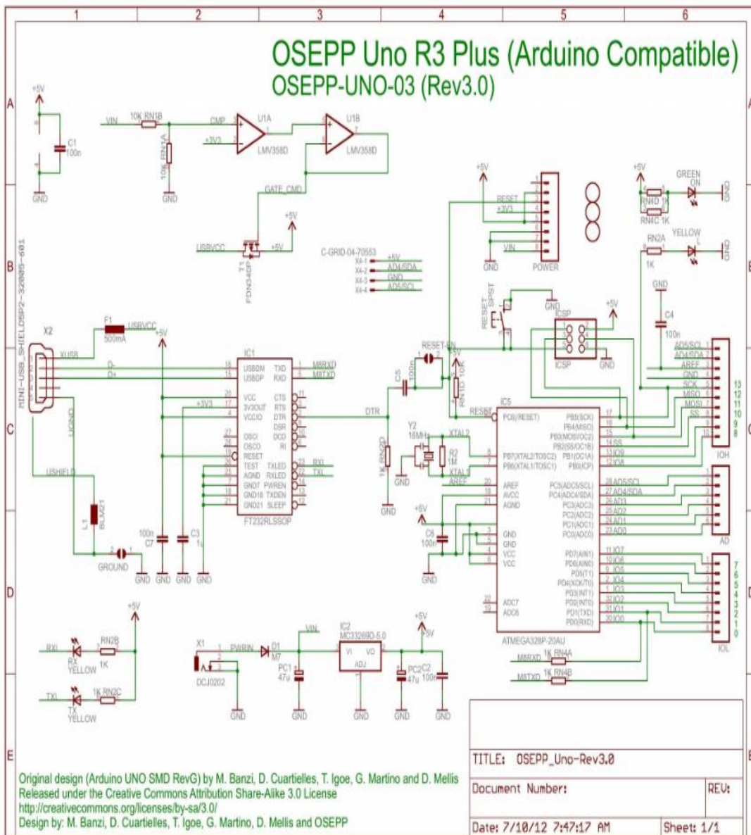
Spesifikasi Arduino Uno wiring setiap komponen
